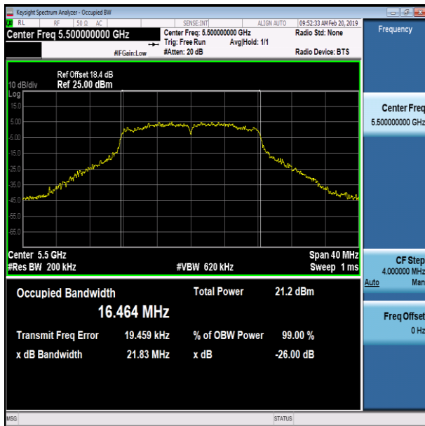
11A-Ant1-5500
