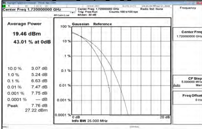
LTE Band66 20MHz 256QAM 100 0 LowCH132072-1720
