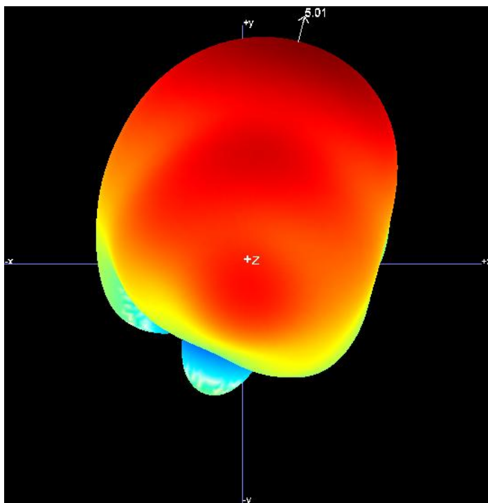
2480MHz
