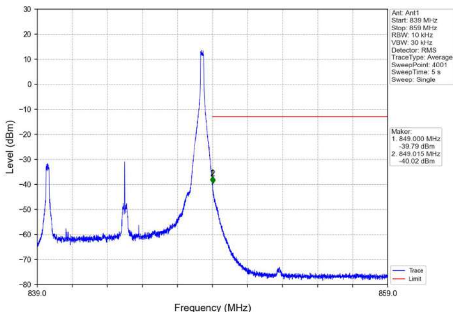
Band26b_10MHz_QPSK_HCH_844MHz_RB_1_49_NTNV
