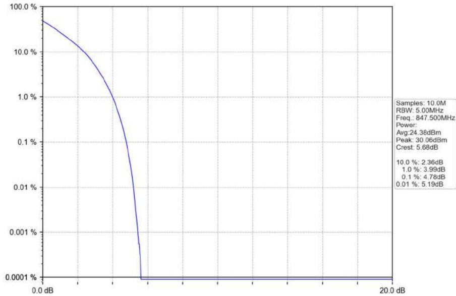
Band26b_3MHz_QPSK_HCH_847.5MHz_RB_15_0_NTNV
