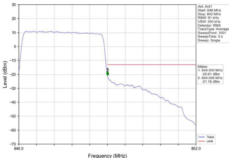
Band26b_3MHz_QPSK_HCH_847.5MHz_RB_15_0_NTNV
