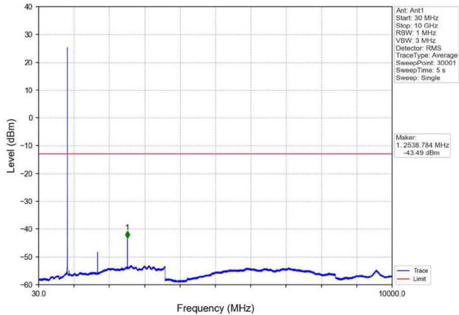
Band26b_3MHz_QPSK_HCH_847.5MHz_RB_1_0_NTNV
