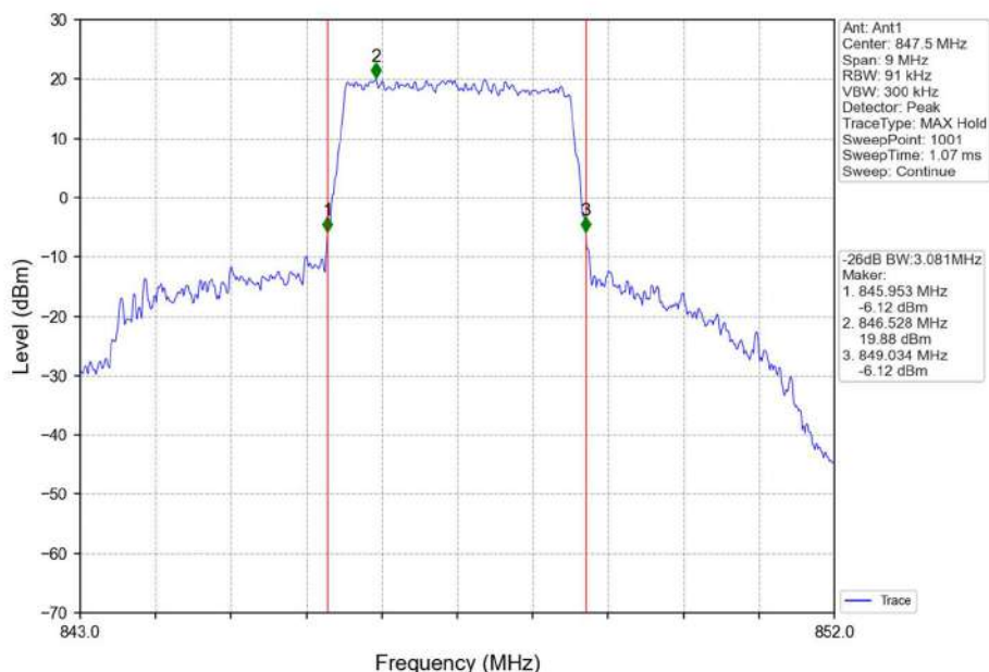
Band26b_3MHz_QPSK_HCH_847.5MHz_RB_15_0_NTNV
