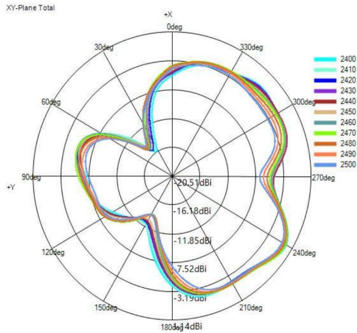
(3) X-Y 面(单位: dBi):
