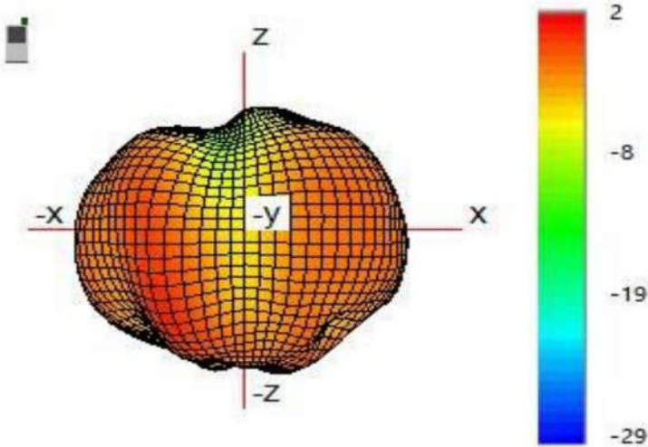
(4) 2.4GHz 的 3D 方向图(单位: dBi):
