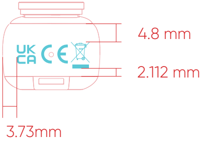
底部视图
