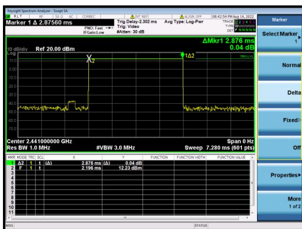
GFSK DH5
