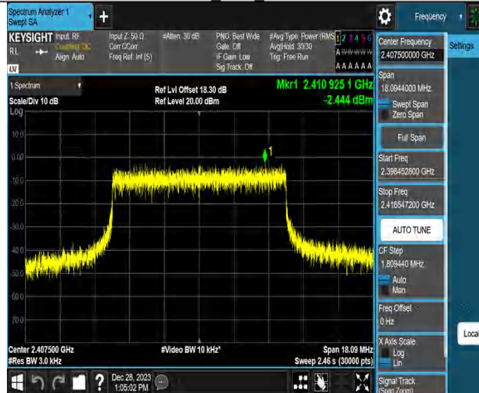
10M_Ant2_2407.5
