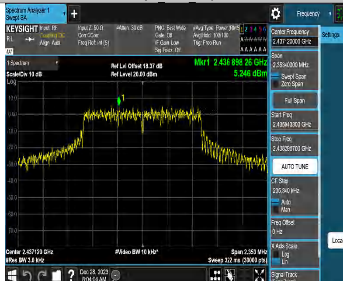
1.4MCA Ant1 2437.12
