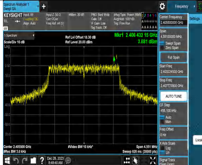
3M_Ant2_2405.5
