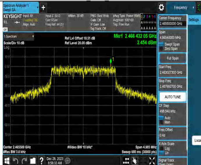
3M_Ant2_2465.5
