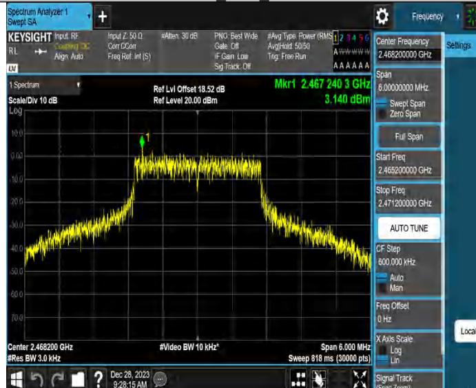
3MCA_Ant2_2468.2
