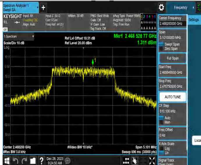
3MCA_Ant2_2468.2
