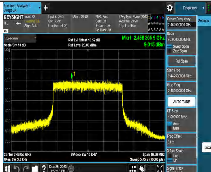
20M_Ant2_2462.5
