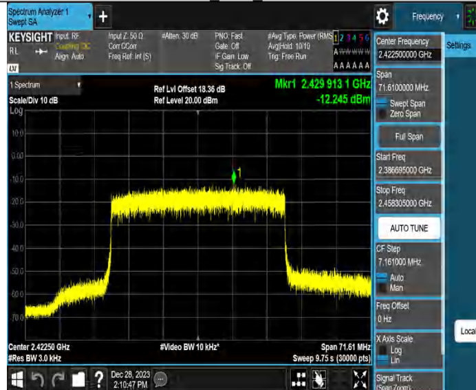
40M_Ant2_2422.5
