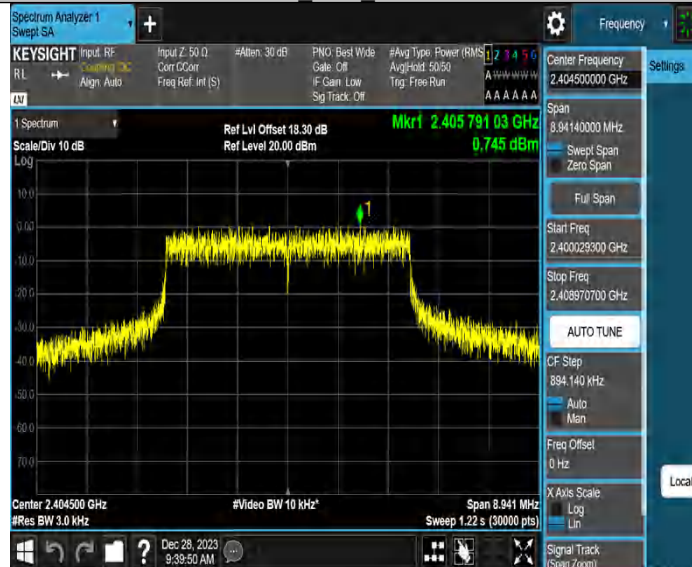
5M_Ant2_2404.5
