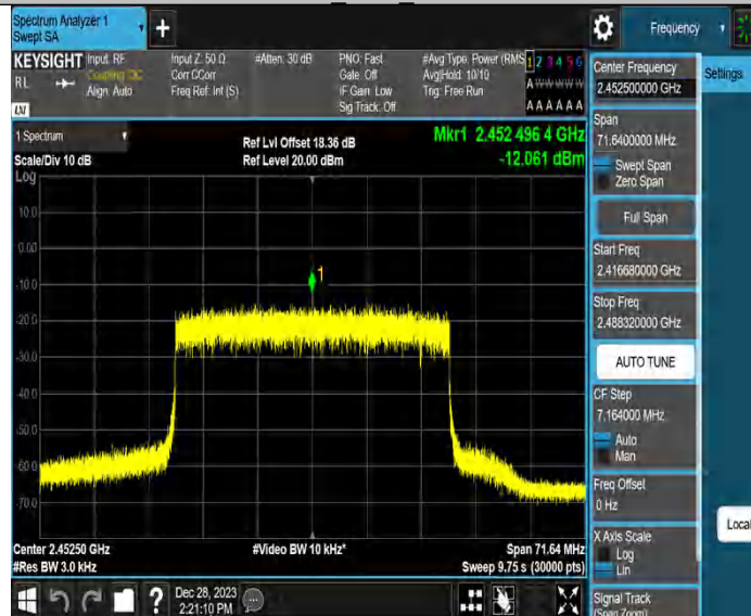
40M_Ant2_2452.5
