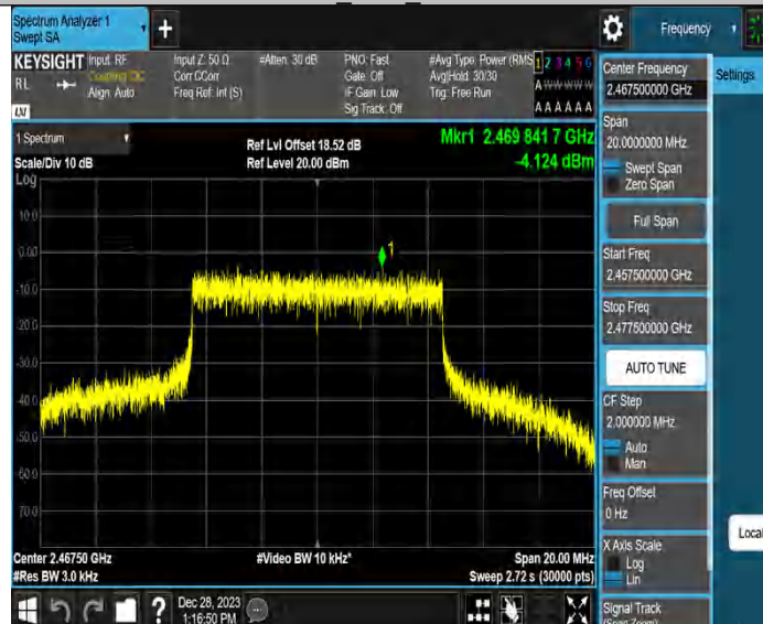
10M_Ant2_2467.5
