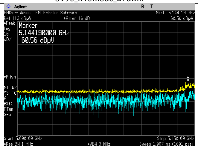
5190_n40mode_peak
