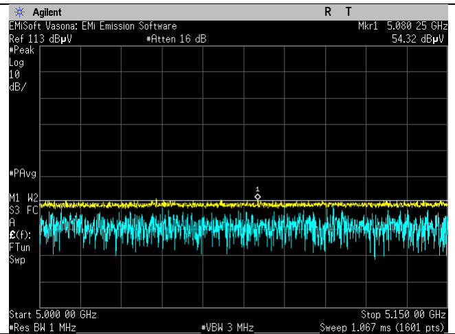
5180_amode_peak
