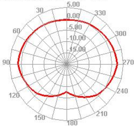
Bluetooth 78 TRP E2
