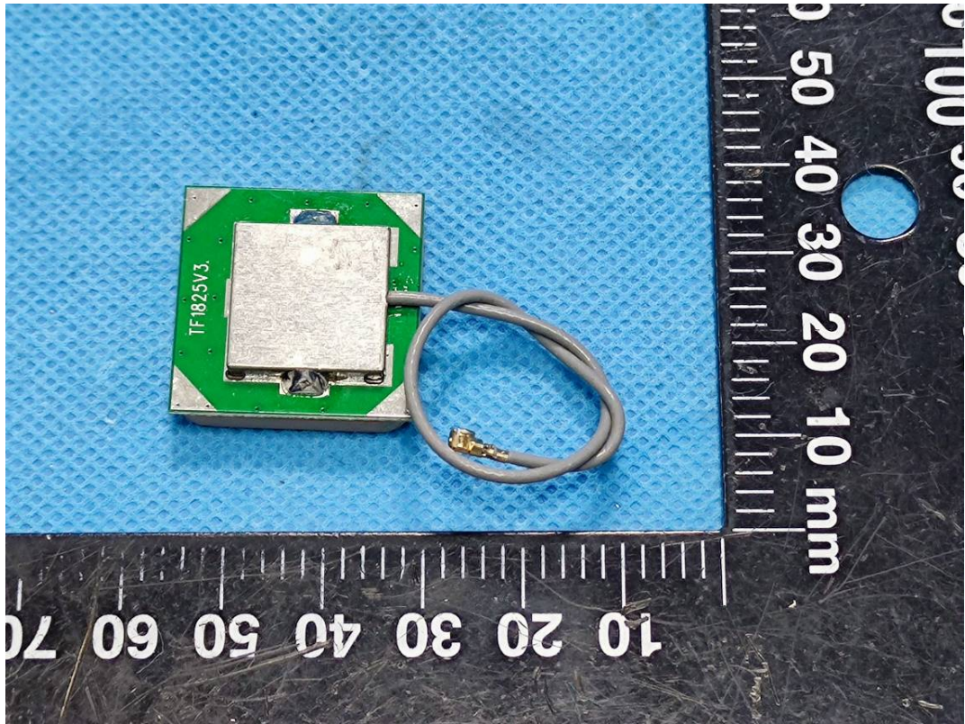
GPS Antenna
