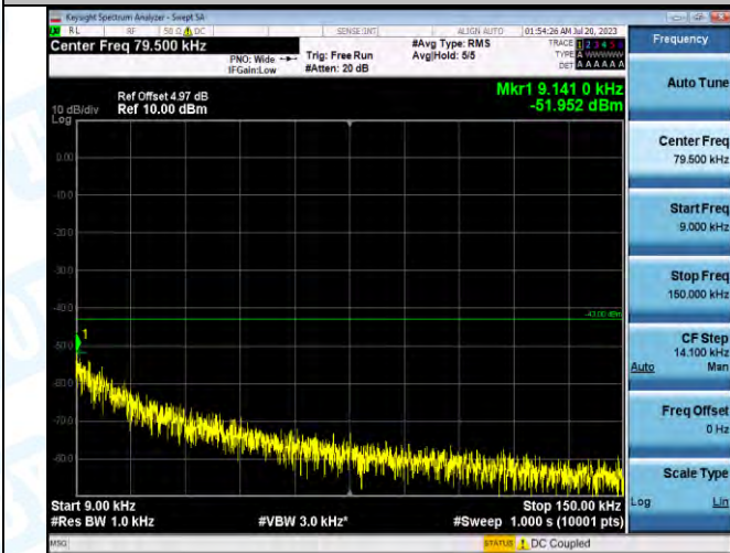
EGPRS1900-810-2-0.009~0.15MHz-PASS
