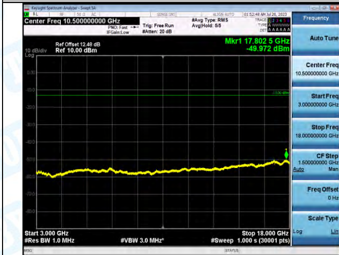
EGPRS1900-512-2-3000~18000MHz-PASS
