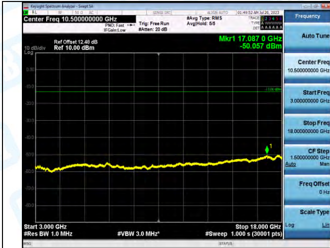
GPRS1900-661-0-3000~18000MHz-PASS
