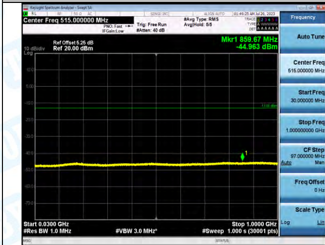
GPRS1900-661-0-30~1000MHz-PASS
