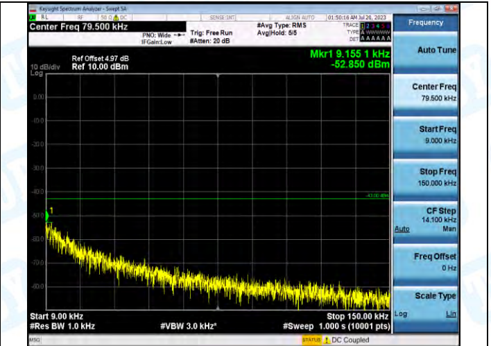
GPRS1900-810-0-0.009~0.15MHz-PASS
