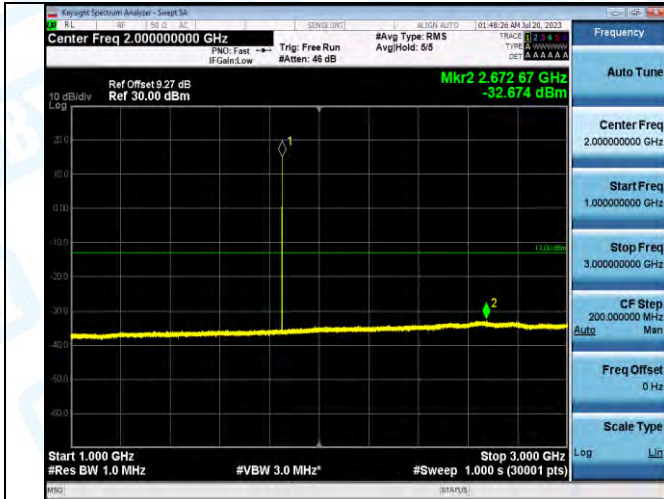
GPRS1900-512-0-1000~3000MHz-PASS
