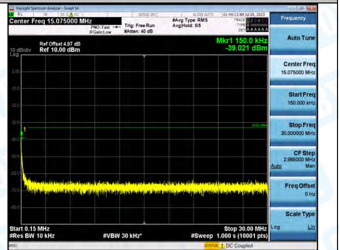
GPRS1900-661-0-0.15~30MHz-PASS
