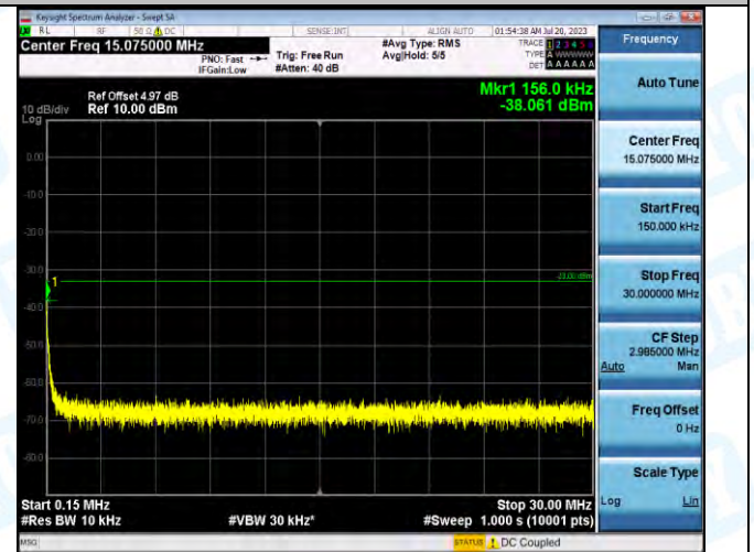
EGPRS1900-810-2-0.15~30MHz-PASS
