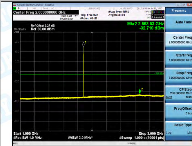
EGPRS1900-661-2-1000~3000MHz-PASS
