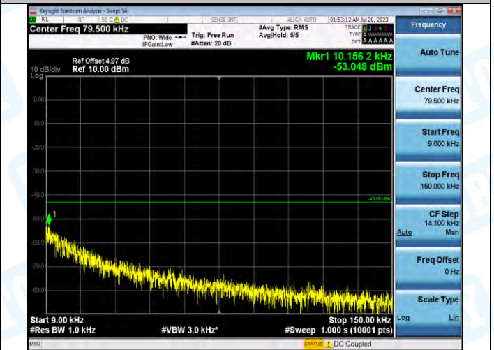
EGPRS1900-661-2-0.009~0.15MHz-PASS
