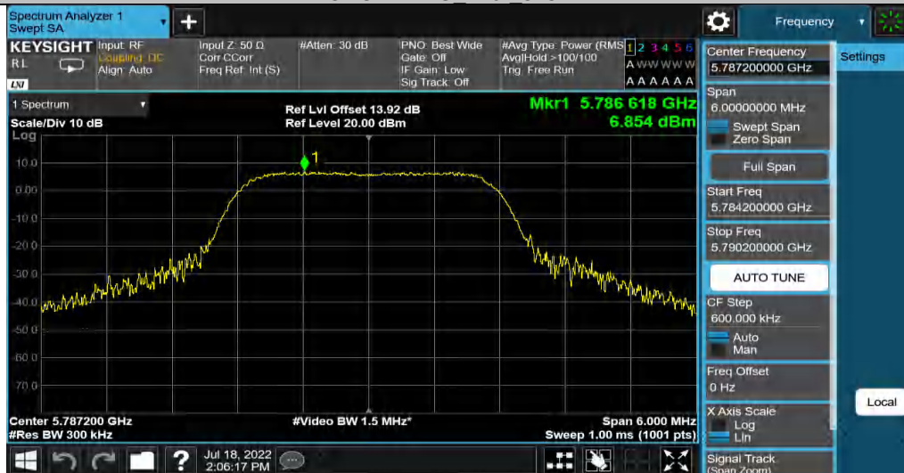
3MCA-MIMO_Ant2_5787.2
