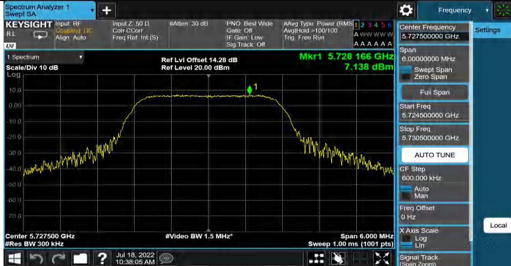
3M-MIMO_Ant2 5727.5
