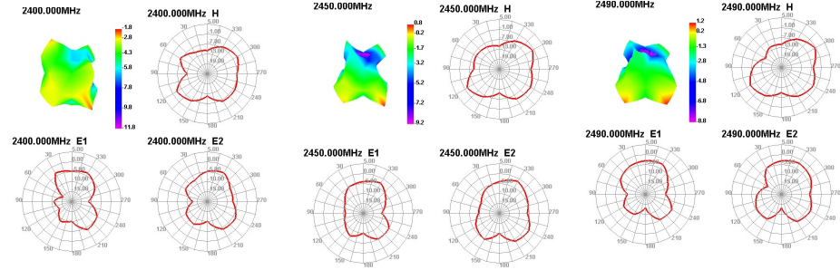
2.4G WIFI天线方向图
