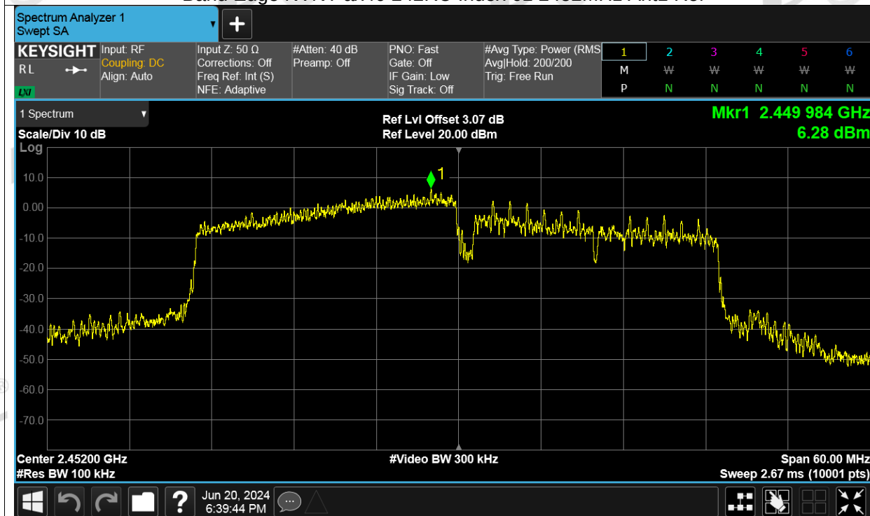
Band Edge NVNT ax40 242RU Index 61 2452MHz Ant1 Emission
