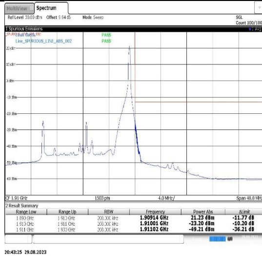
Band2-20MHz-QPSK-18700-1RB#0
