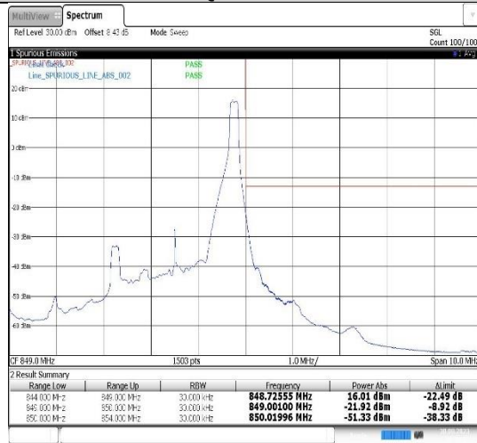
Band5-3MHz-QPSK-20635-1RB#14
