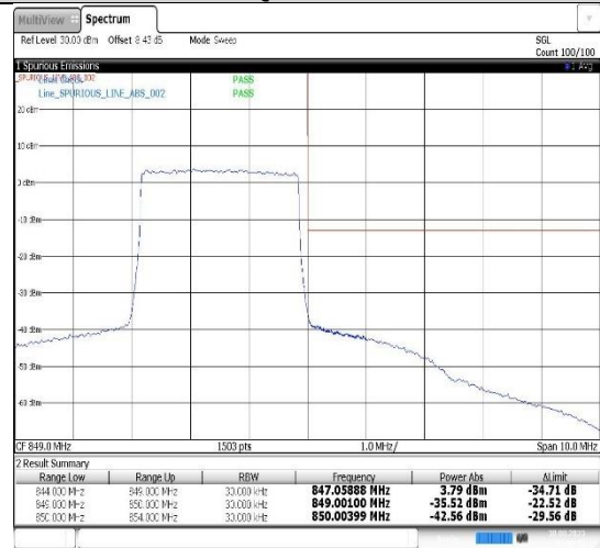
Band5-3MHz-QPSK-20635-15RB#0
