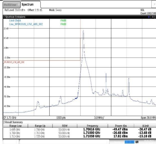
Band4-10MHz-QPSK-20000-1RB#0
