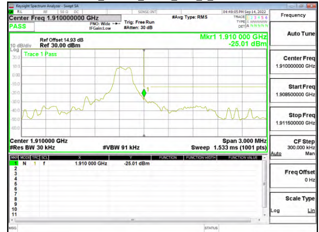
Band2_1.4MHz_QPSK_RB1_5_CH19193
