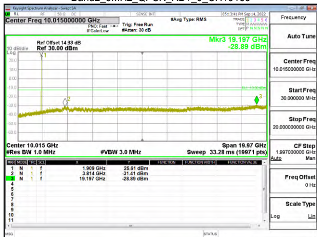
Band2_3MHz_QPSK_RB1_0_CH19185
