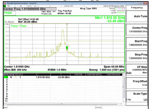
Band2_20MHz_QPSK_RB1_5_CH19100
