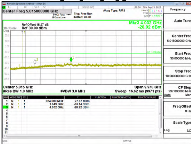
Band5_3MHz_QPSK_RB1_0_CH20525
