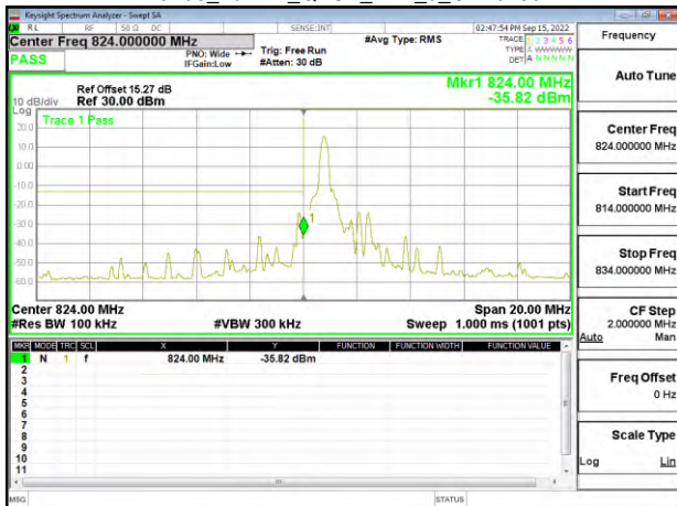
Band5_10MHz_QPSK_RB1_0_CH20450
