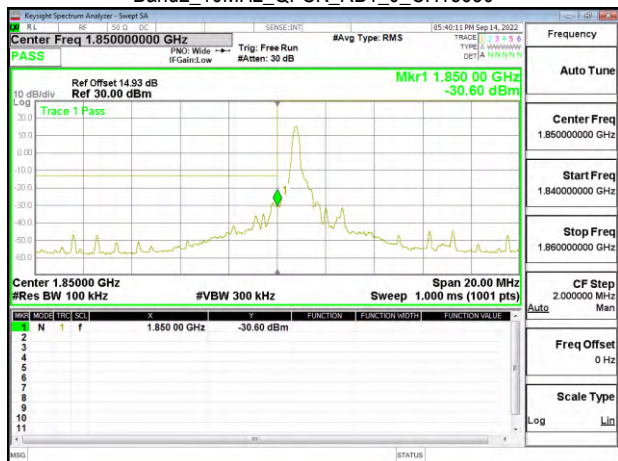
Band2_10MHz_QPSK_RB1_0_CH18650
