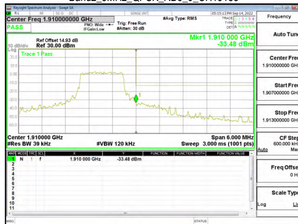
Band2_3MHz_QPSK_RB6_0_CH19185
