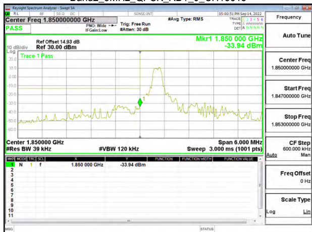
Band2_3MHz_QPSK_RB1_0_CH18615
