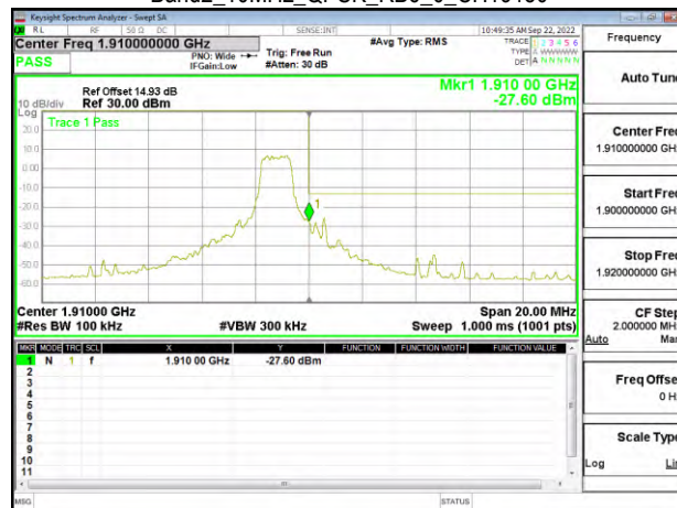
Band2_10MHz_QPSK_RB6_0_CH19150
