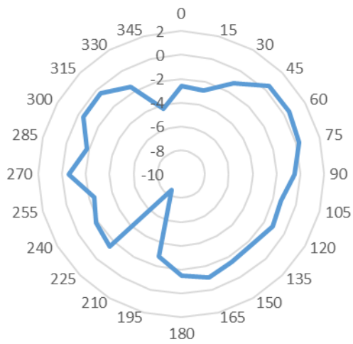
5.75GHz
