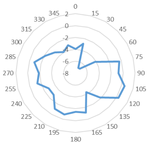
5.25GHz
