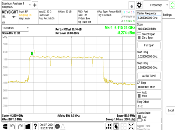
802.11be_320MHz_Chain1_6265MHz_3x996_MRU4
