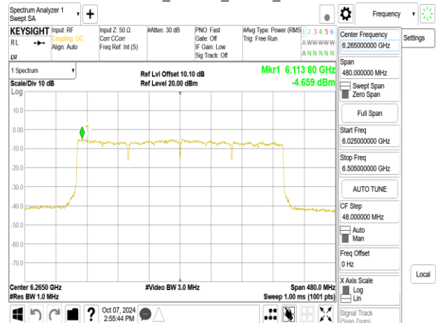
802.11be_320MHz_Chain1_6265MHz
