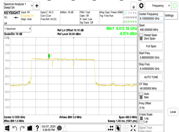
802.11be_320MHz_Chain0_6105MHz_RU996x2+484_Punc40
