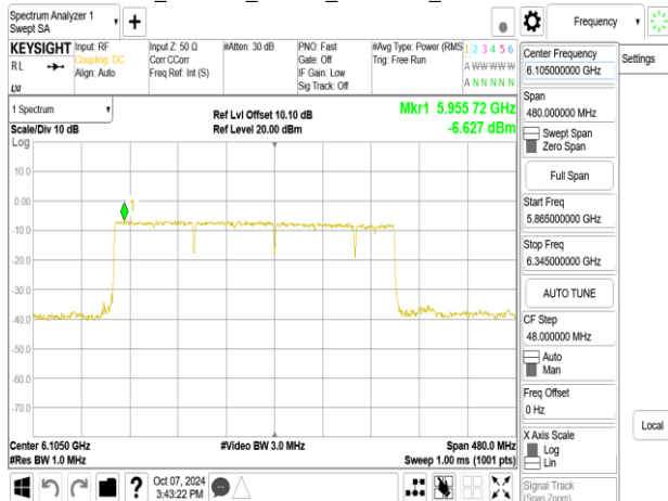
802.11be_320MHz_Chain0_6105MHz_3x996+484_MRUA
