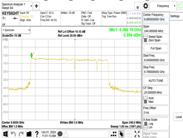
802.11be_160MHz_Chain1_6665MHz_RU996_67
