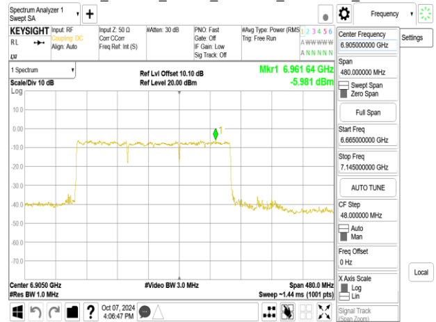
802.11be_320MHz_Chain1_6905MHz_RU996x2+484_Punc40
