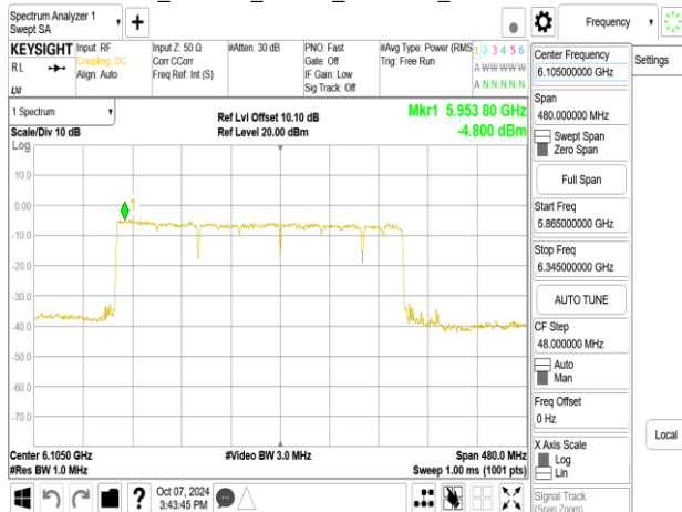
802.11be_320MHz_Chain1_6105MHz_3x996+484_MRU8
