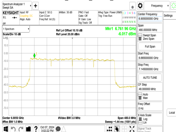
802.11be_320MHz_Chain1_6905MHz_2x996+484 MRU6
