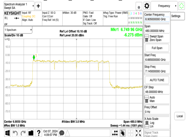
802.11be_320MHz_Chain1_6905MHz_3x996+484 MRU1
