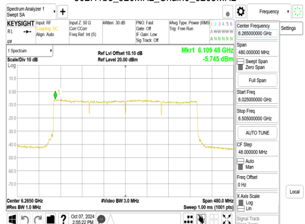
802.11be_320MHz_Chain0_6265MHz
