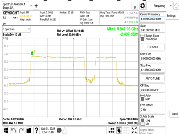
802.11be_160MHz_Chain1_6025MHz_996+484_MRU2
