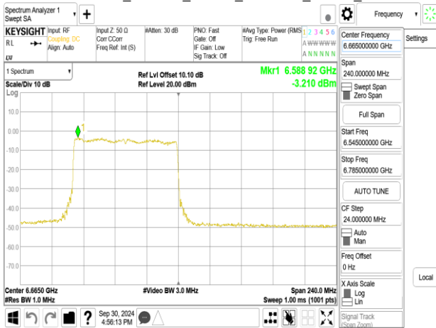
802.11be_160MHz_Chain1_6665MHz_RU996_S67
