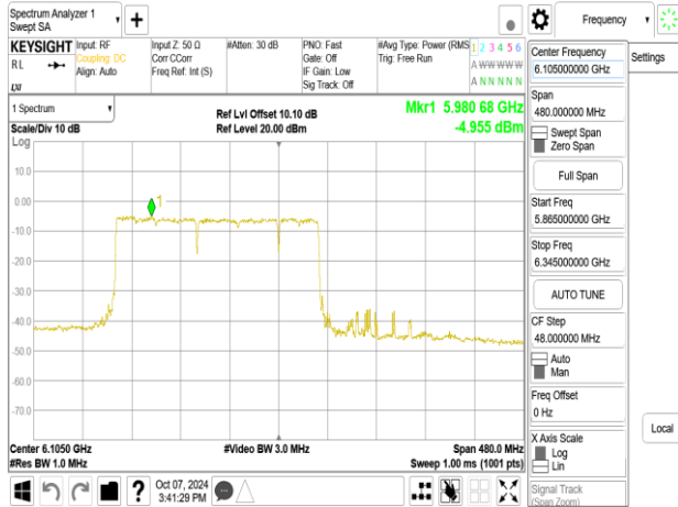
802.11be_320MHz_Chain1_6105MHz_3x996+484_MRU8
