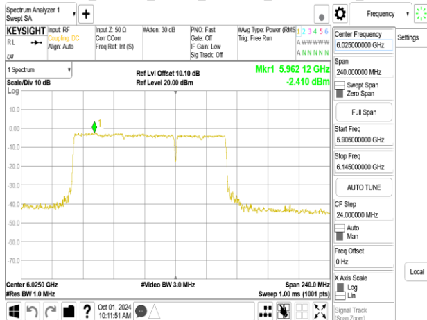
802.11be_160MHz_Chain1_6025MHz_996+484_MRU2
