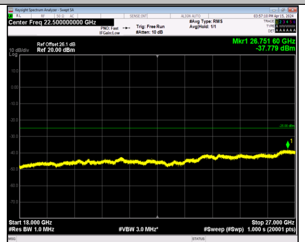
Band7_20MHz_QPSK_21350_1RB#0_18000~27000_18000~27000
