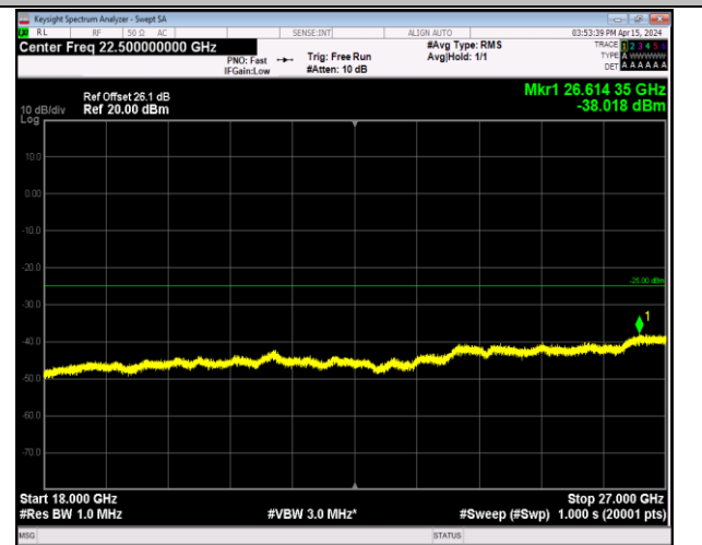
Band7_20MHz_QPSK_20850_1RB#0_18000~27000_18000~27000
