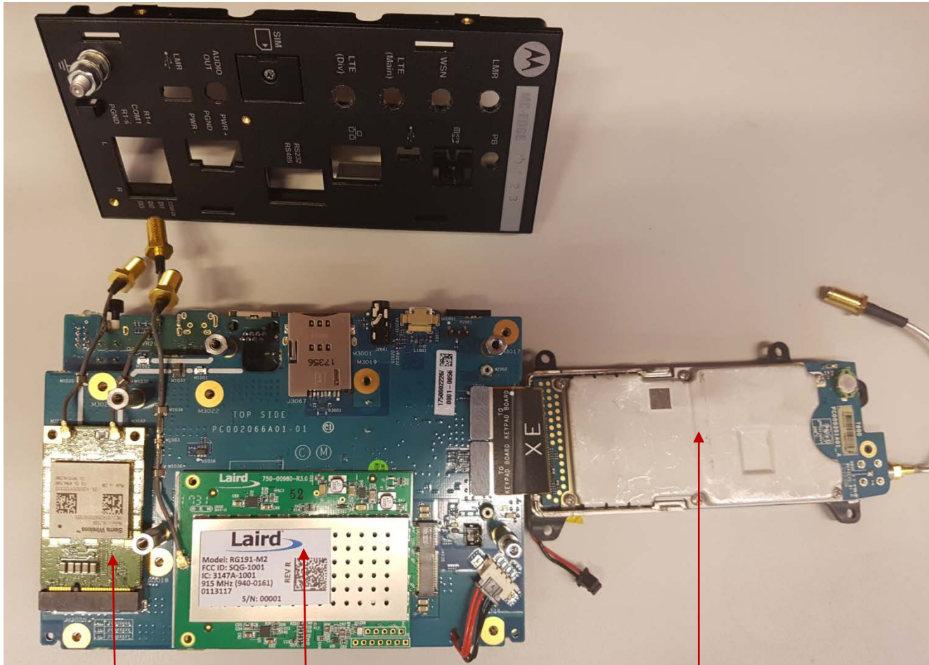
LTE Module
