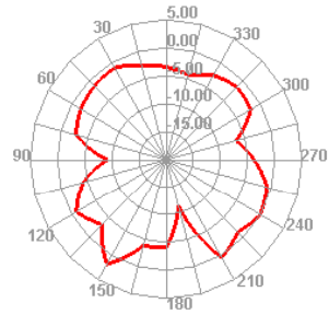
2410.000MHz E2
