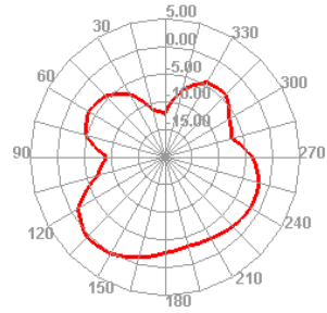
2410.000MHz H
