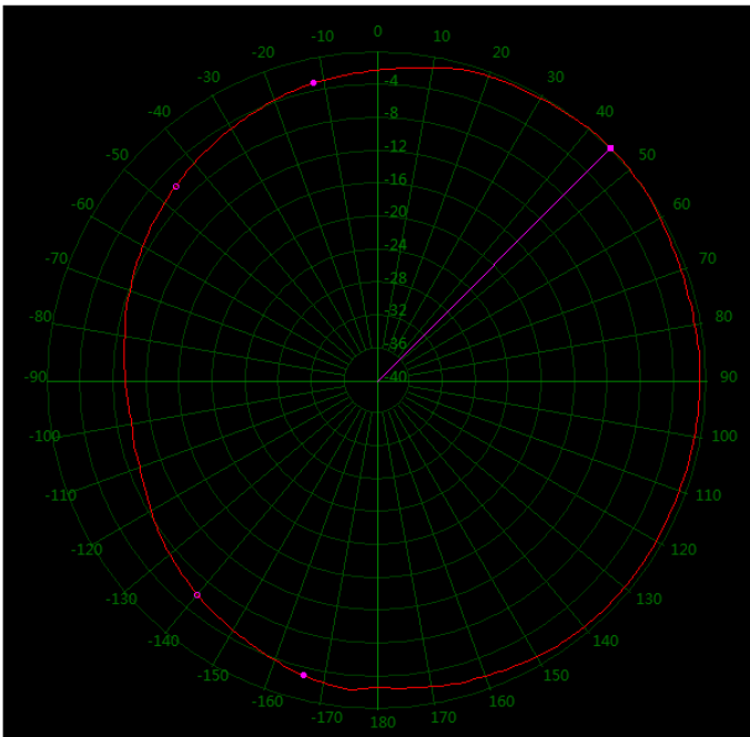
158 MHz Horizontal 360°
