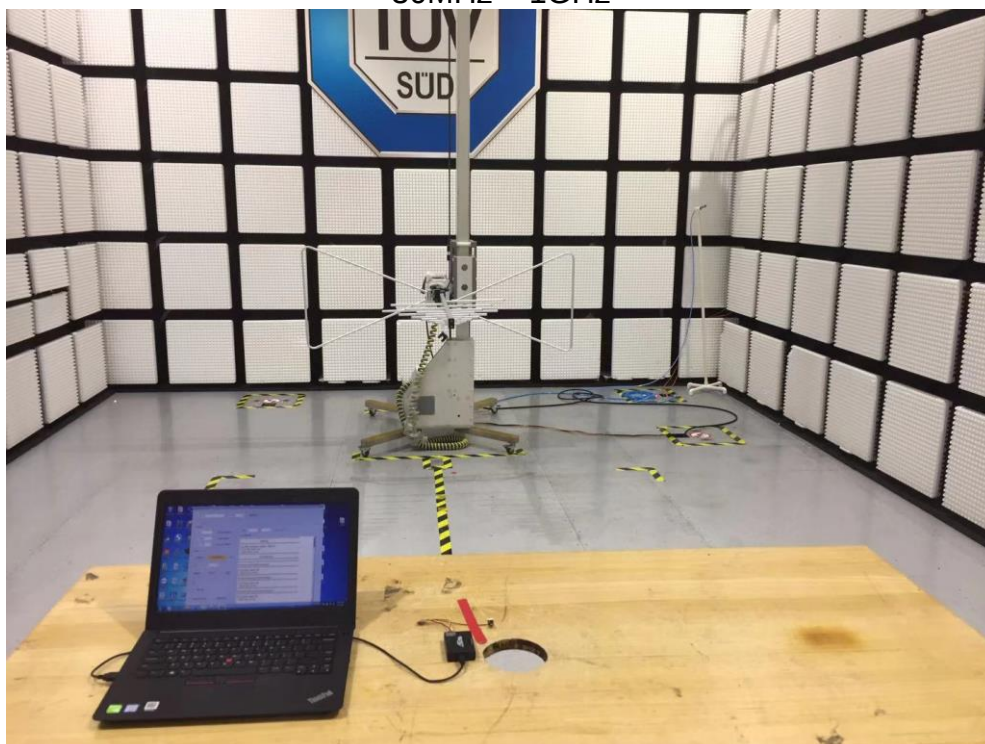
30MHz ~ 1GHz
