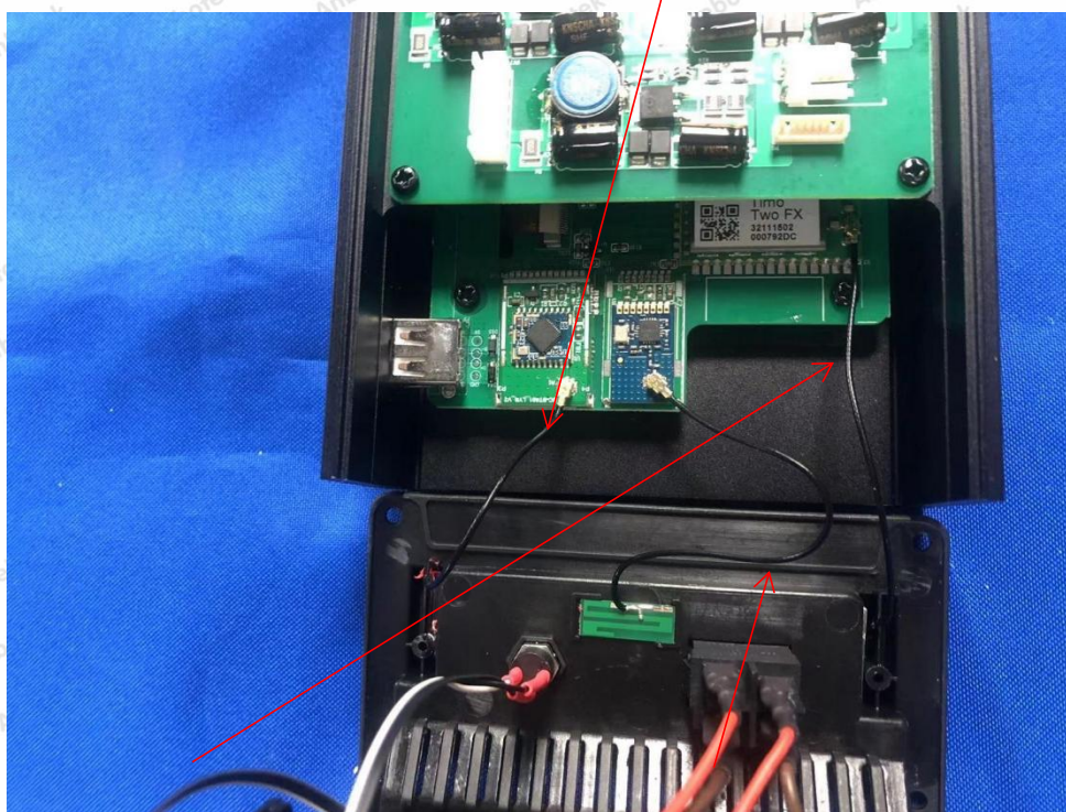
Lumenradio ANT
