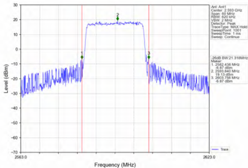
Band41_20MHz_QPSK_MCH_2593MHz_RB_100_0_NTNV
