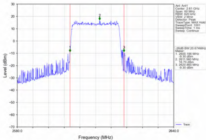
Band38_20MHz_256QAM_HCH_2610MHz_RB_100_0_NTNV
