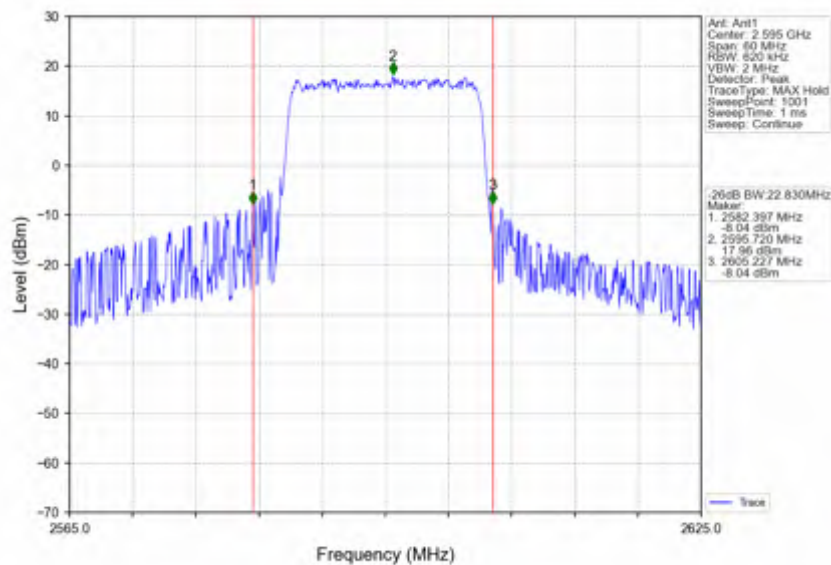
Band38_20MHz_QPSK_MCH_2595MHz_RB_100_0_NTNV
