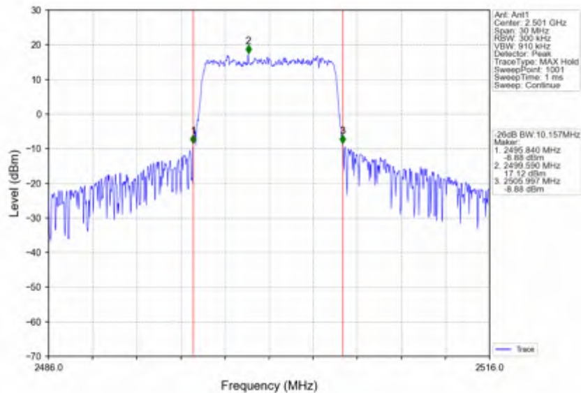
Band41_10MHz_256QAM_LCH_2501MHz_RB_50_0_NTNV
