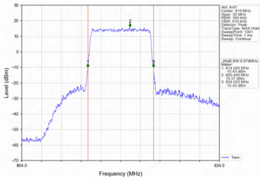
Band26a 10MHz 16QAM HCH 819MHz RB 50 0 NTNV
