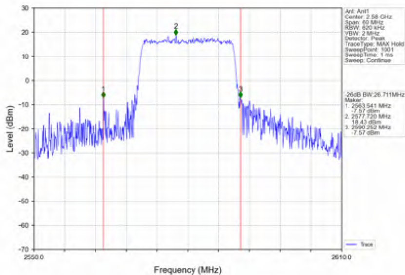
Band38_20MHz_16QAM_LCH_2580MHz_RB_100_0_NTNV
