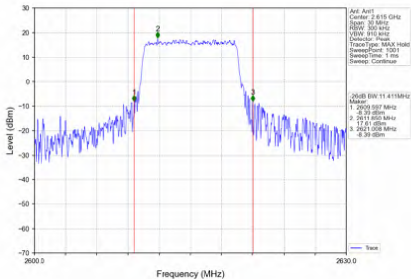
Band38 10MHz 16QAM HCH 2615MHz RB 50 0 NTNV
