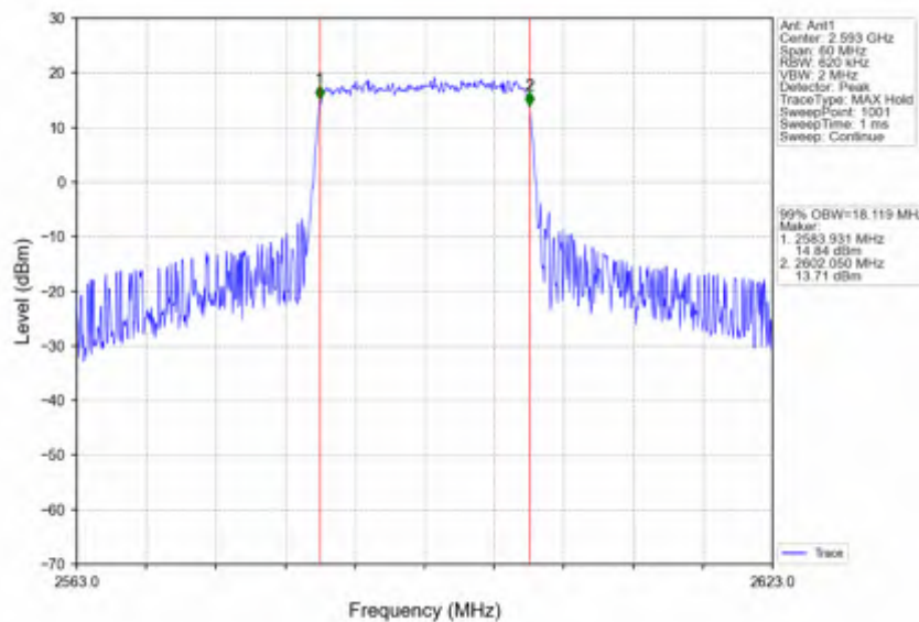
Band41_20MHz_QPSK_MCH_2593MHz_RB_100_0_NTNV
