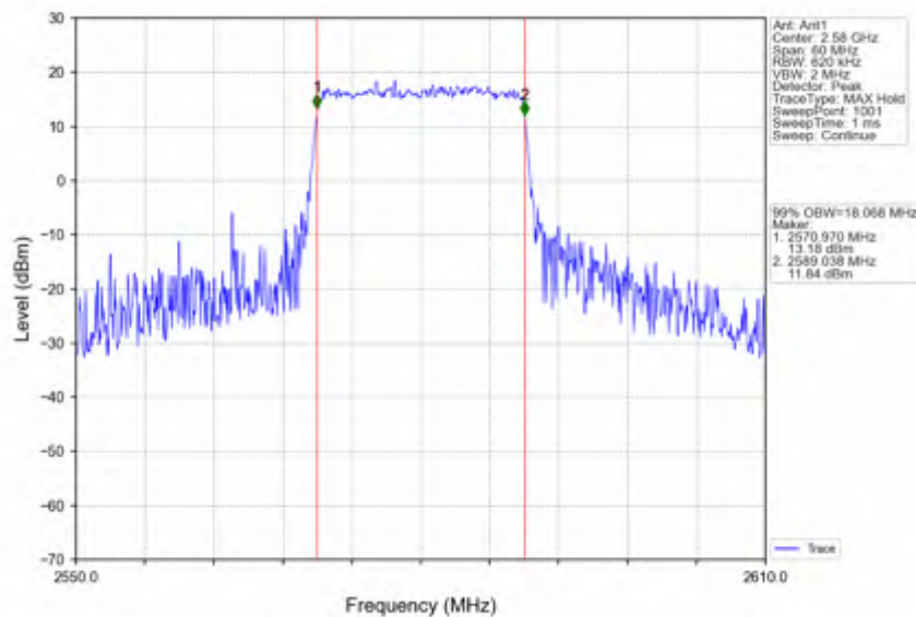
Band38_20MHz_16QAM_LCH_2580MHz_RB_100_0_NTNV
