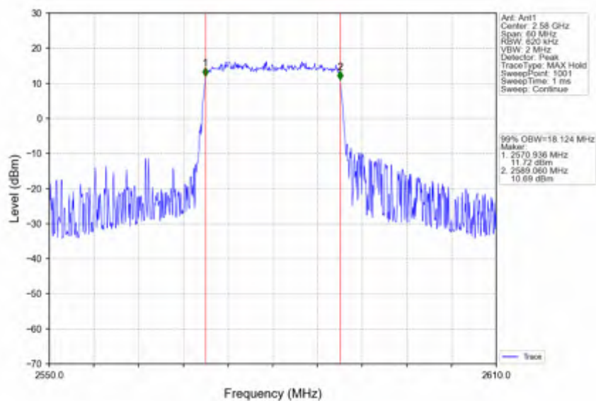
Band38 20MHz 256QAM LCH 2580MHz RB 100 0 NTNV
