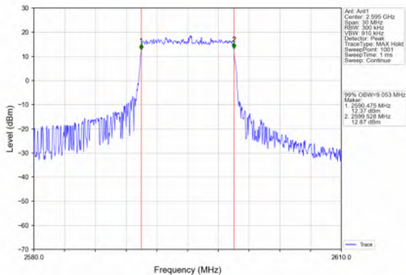
Band38 10MHz 64QAM MCH 2595MHz RB 50 0 NTNv
