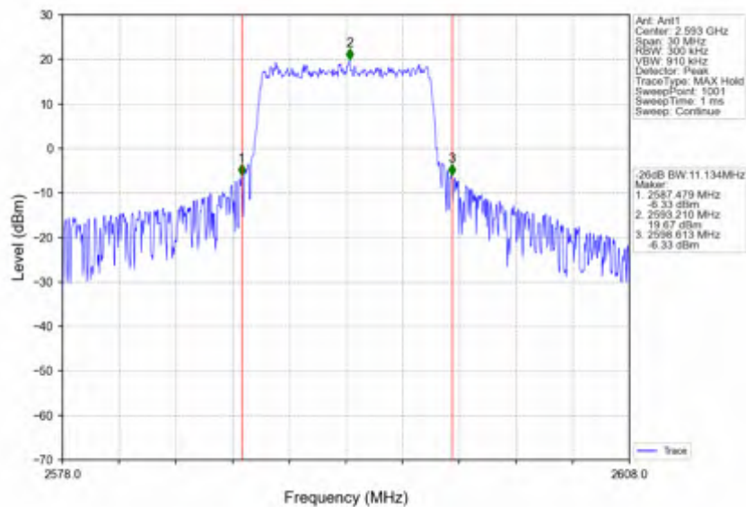
Band41_10MHz_QPSK_MCH_2593MHz_RB_50_0_NTNV
