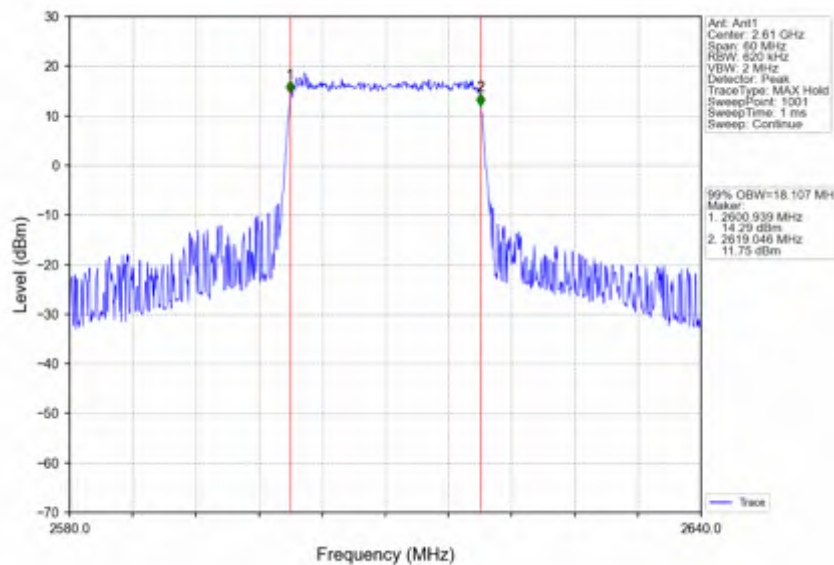
Band38_20MHz_16QAM_HCH_2610MHz_RB_100_0_NTNV
