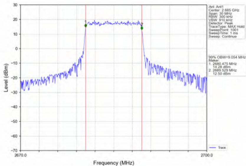
Band41_10MHz_16QAM_HCH_2685MHz_RB_50_0_NTNV
