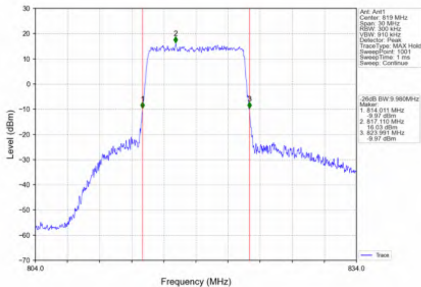
Band26a_10MHz_QPSK_MCH_819MHz_RB_50_0_NTNV
