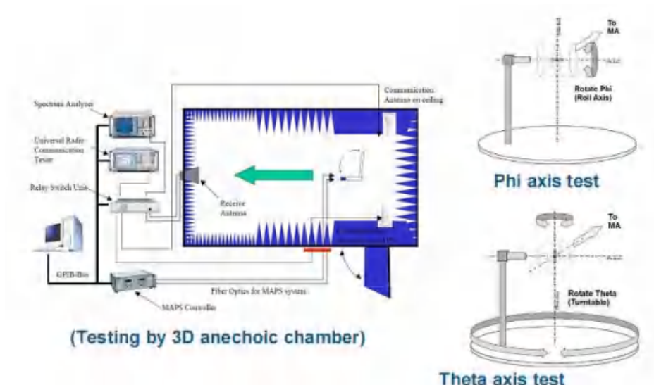
图 1 Test topology
