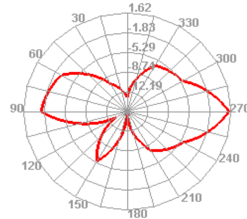
2500.000MHz E1
