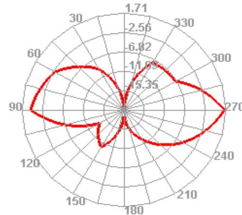
2400.000MHz E1
