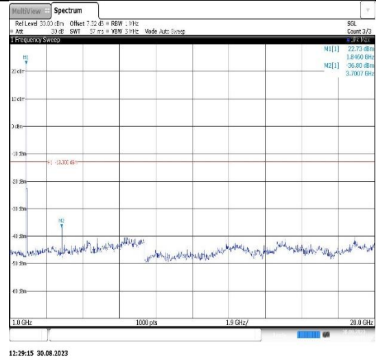
Band25-20MHz-16QAM-26365-1RB#0- Range2:1000~20000MHz
