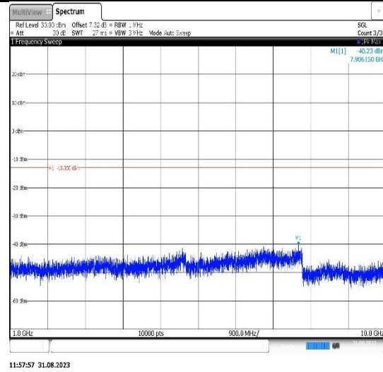
Band26(824-849)-1.4MHz-QPSK-26915-1RB#0-Range2:1000~10000MHz
