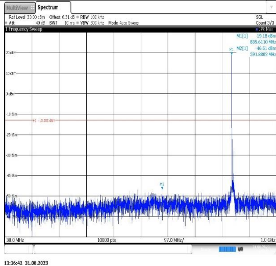
Band26(824-849)-15MHz-QPSK-26865-1RB#0- Range1:30~1000MHz
