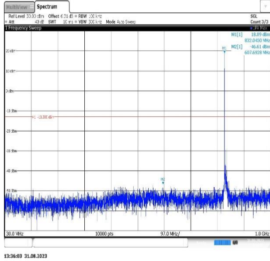
Band26(824-849)-10MHz-16QAM-26990-1RB#0- Range1:30~1000MHz
