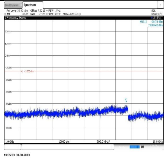
Band26(824-849)-10MHz-16QAM-26915-1RB#0- Range2:1000~10000MHz
