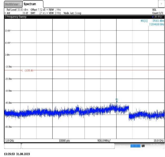
Band26(824-849)-10MHz-QPSK-26990-1RB#0-Range2:1000~10000MHz
