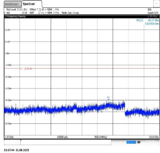
Band26(824-849)-5MHz-QPSK-27015-1RB#0-Range2:1000~10000MHz
