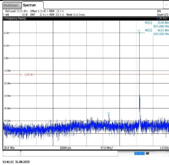
Band26(824-849)-3MHz-QPSK-26915-1RB#0-Range1:30~1000MHz
