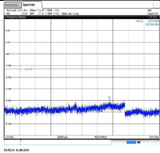
Band26(824-849)-10MHz-QPSK-26915-1RB#0-Range2:1000~10000MHz
