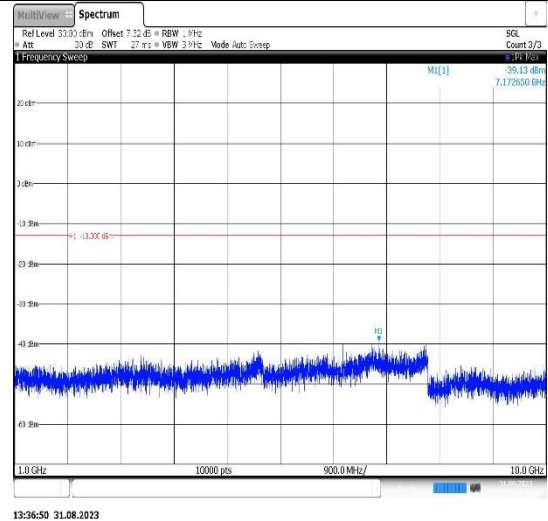
Band26(824-849)-15MHz-QPSK-26865-1RB#0- Range2:1000~10000MHz
