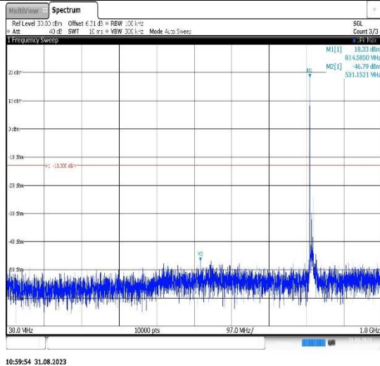
Band26(824-849)-1.4MHz-QPSK-26797-1RB#0-Range1:30~1000MHz
