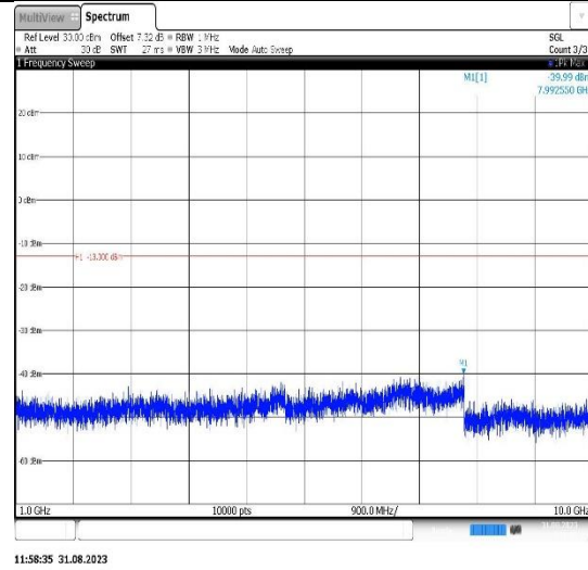
Band26(824-849)-1.4MHz-QPSK-27033-1RB#0-Range2:1000~10000MHz
