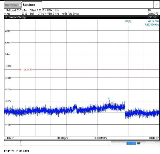
Band26(824-849)-3MHz-QPSK-26915-1RB#0-Range2:1000~10000MHz
