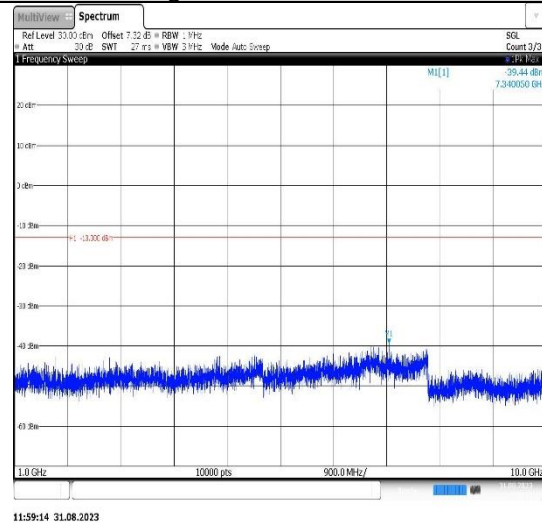
Band26(824-849)-1.4MHz-16QAM-26797-1RB#0-Range2:1000~10000MHz
