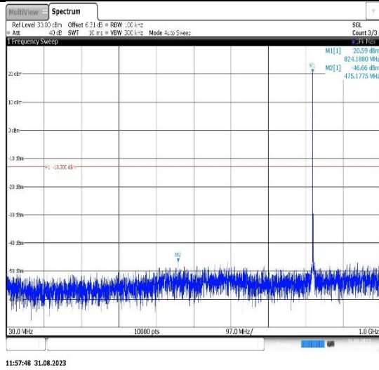
Band26(824-849)-1.4MHz-QPSK-26915-1RB#0-Range1:30~1000MHz
