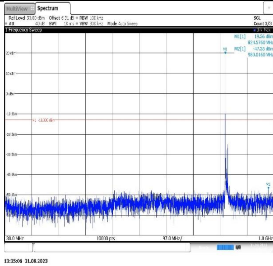
Band26(824-849)-10MHz-QPSK-26915-1RB#0-Range1:30~1000MHz
