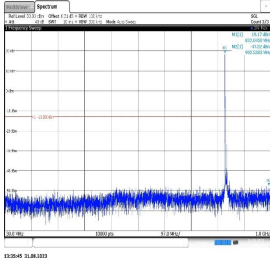
Band26(824-849)-10MHz-QPSK-26990-1RB#0-Range1:30~1000MHz
