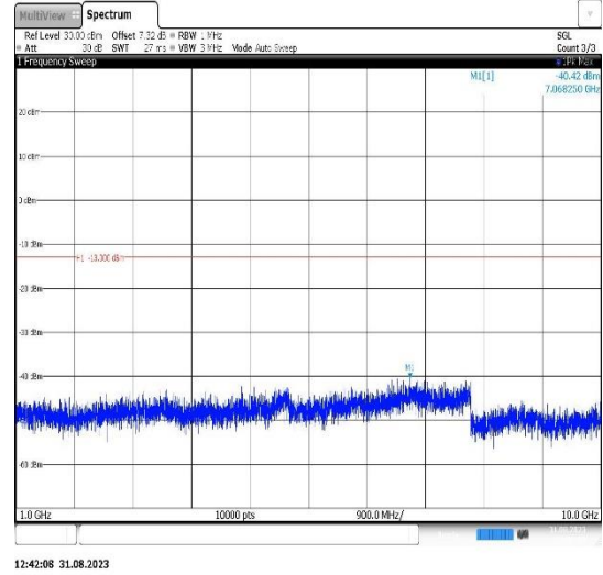
Band26(824-849)-3MHz-QPSK-27025-1RB#0-Range2:1000~10000MHz
