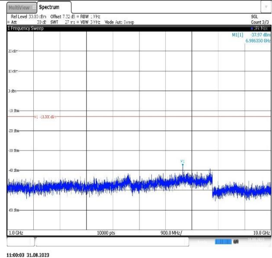
Band26(824-849)-1.4MHz-QPSK-26797-1RB#0-Range2:1000~10000MHz
