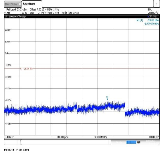
Band26(824-849)-10MHz-16QAM-26990-1RB#0- Range2:1000~10000MHz
