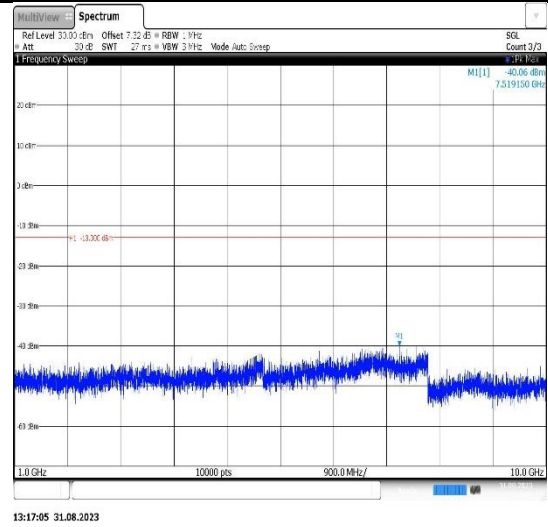
Band26(824-849)-5MHz-QPSK-26915-1RB#0-Range2:1000~10000MHz
