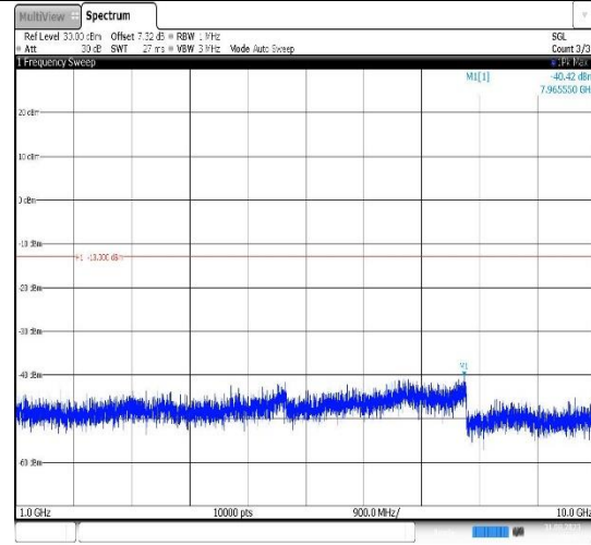
Band26(824-849)-3MHz-16QAM-27025-1RB#0-Range2:1000~10000MHz
