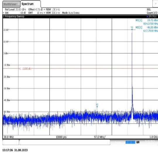
Band26(824-849)-5MHz-QPSK-27015-1RB#0-Range1:30~1000MHz
