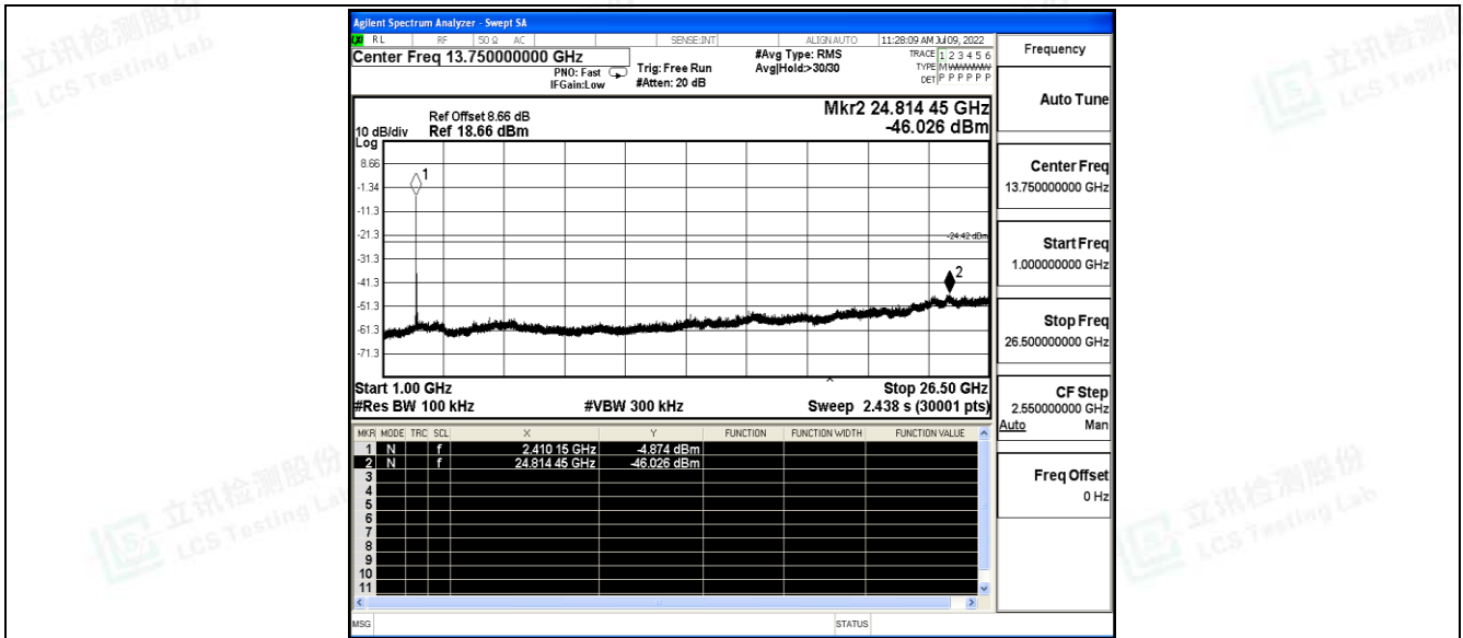
11B_Ant0_2437_0~Reference
