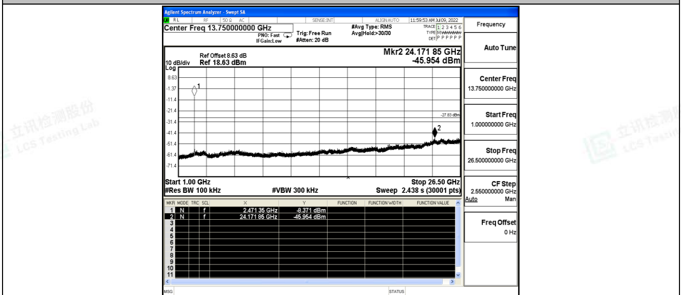
11G_Ant0_2412_0-Reference
