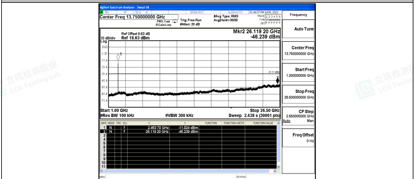
11AX40SISO_Ant0_2422_0-Reference
