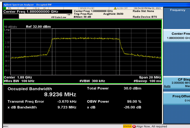
Band2-10MHz-QPSK-18900-50RB#0-8.9236
