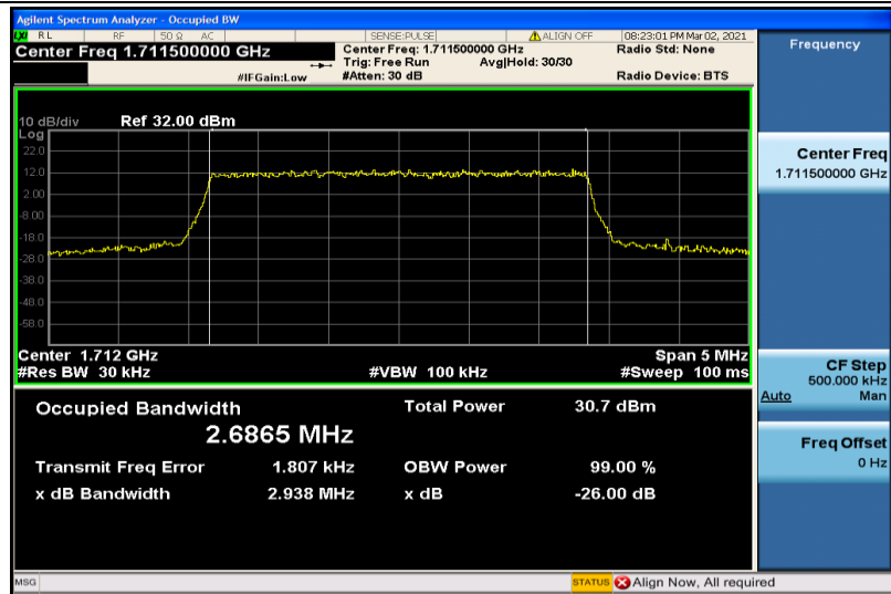
Band4-3MHz-QPSK-19965-15RB#0-2.6865
