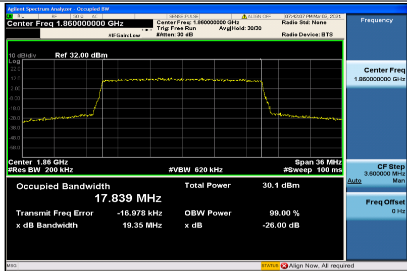
Band2-20MHz-QPSK-18700-100RB#0-17.839
