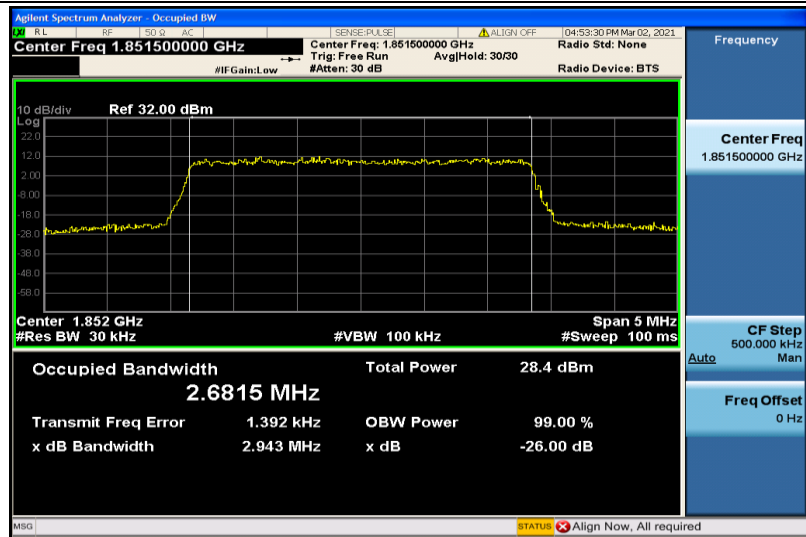
Band2-3MHz-16QAM-18615-15RB#0-2.6815
