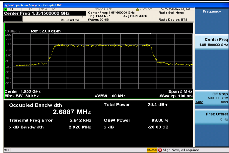
Band2-3MHz-QPSK-18615-15RB#0-2.6887
