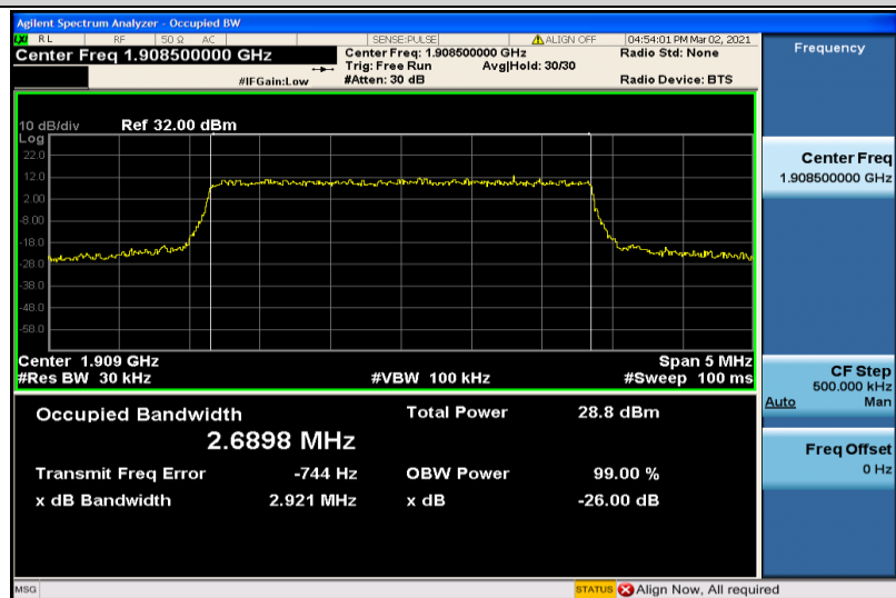
Band2-3MHz-QPSK-19185-15RB#0-2.6898
