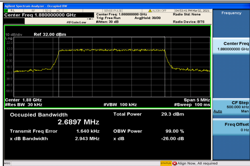
Band2-3MHz-QPSK-18900-15RB#0-2.6897
