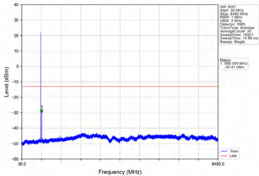
Band5_10MHz_QPSK_HCH_844MHz_RB_1_49_NTNV
