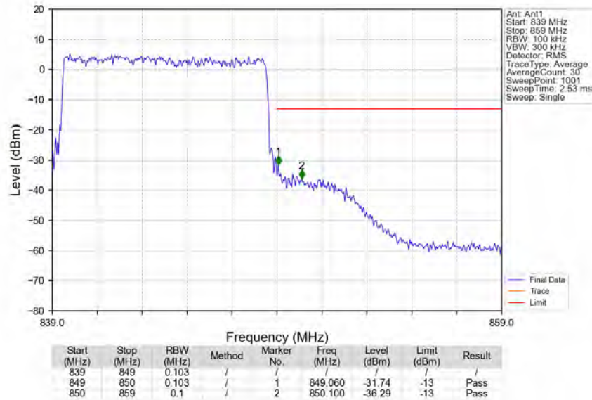
Band5_10MHz_QPSK_HCH_844MHz_RB_50_0_NTNV
