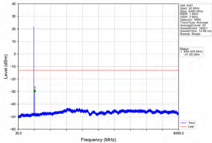
Band5_3MHz_QPSK_HCH_847.5MHz_RB_1_14_NTNV
