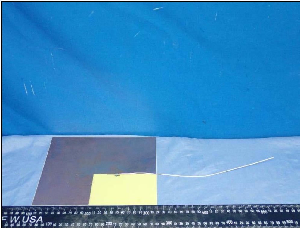
Antenna 2 (Brand: Hong-Bo / Model: 260-25083)
