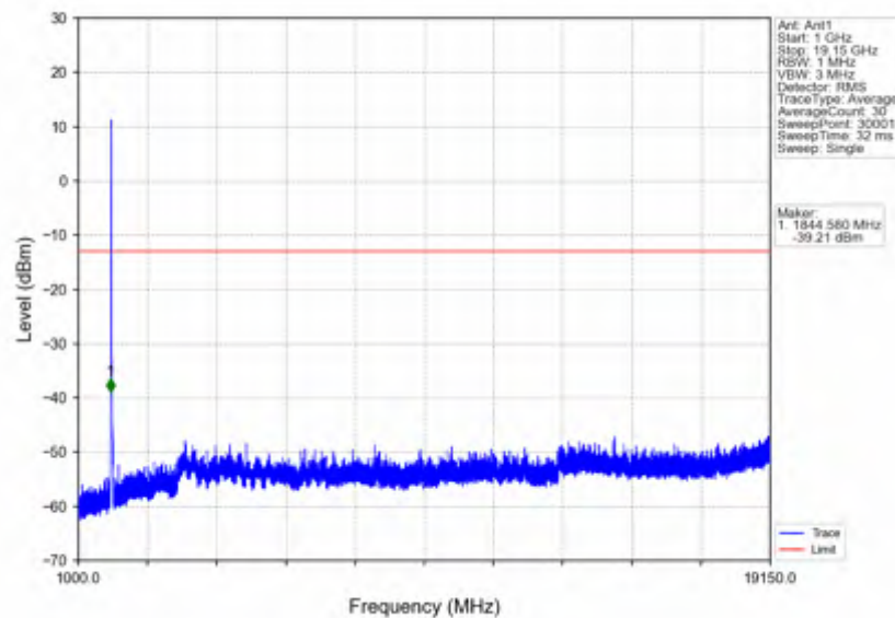
n25_30kHz_SISO_NTNV_20MHz_DFT-s-OFDM QPSK_1860MHz_Inner_1RB_Left
