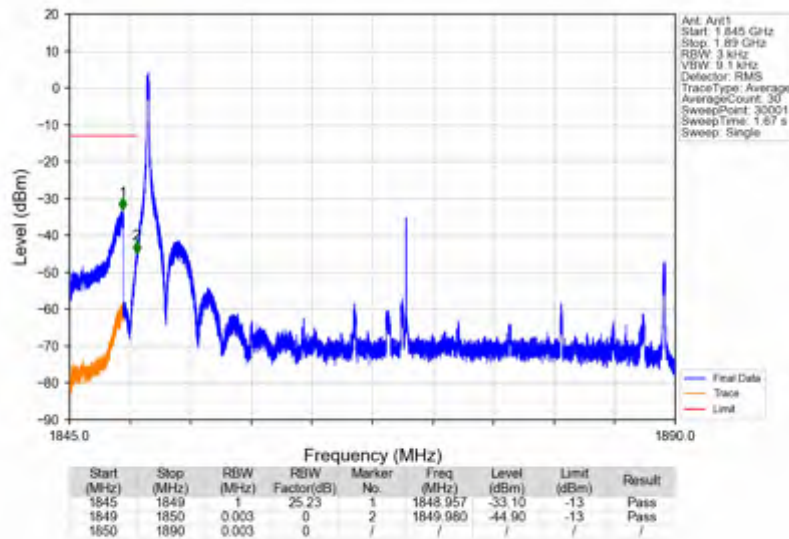
n25_15kHz_SISO_NTNV_40MHz_DFT-s-OFDM QPSK_1870MHz_Inner_1RB_Left
