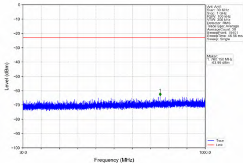
n25_15kHz_SISO_NTNV_40MHz_DFT-s-OFDM QPSK_1870MHz_Inner_1RB_Left
