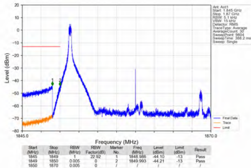
n25_30kHz_SISO_NTNV_20MHz_DFT-s-OFDM QPSK_1860MHz_Inner_1RB_Left
