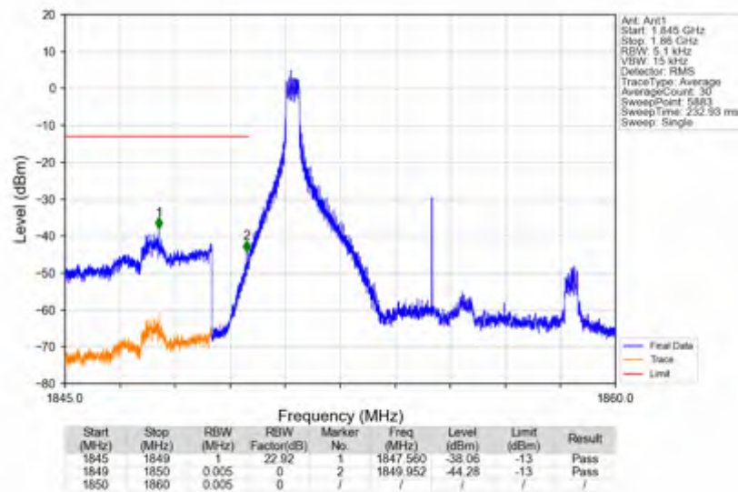
n25_30kHz_SISO_NTNV_10MHz_DFT-s-OFDM QPSK_1855MHz_Inner_1RB_Left
