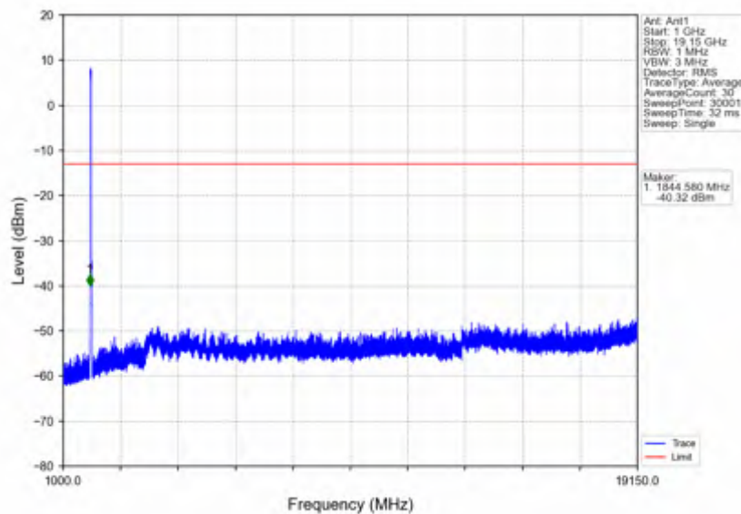
n25_15kHz_SISO_NTNV_40MHz_DFT-s-OFDM QPSK_1870MHz_Inner_1RB_Left
