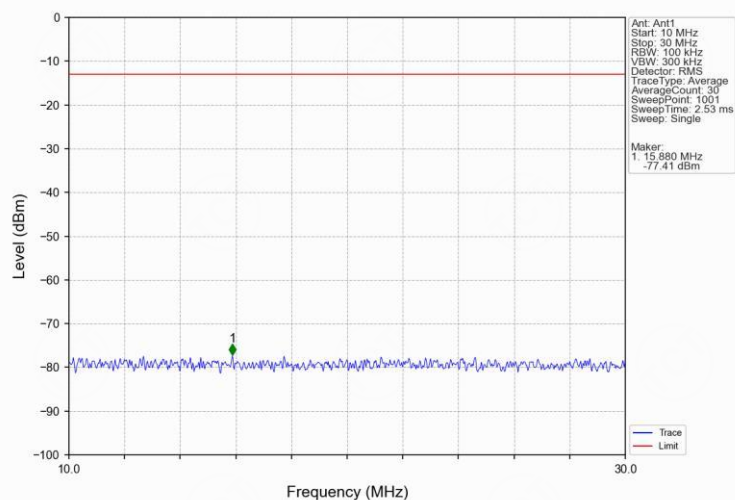
Band26b_3MHz_QPSK_HCH_847.5MHz_RB_1_0_NTNV
