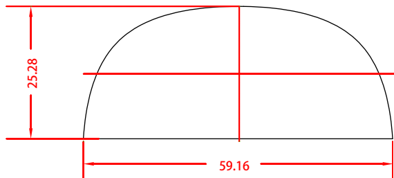
结构尺寸图
