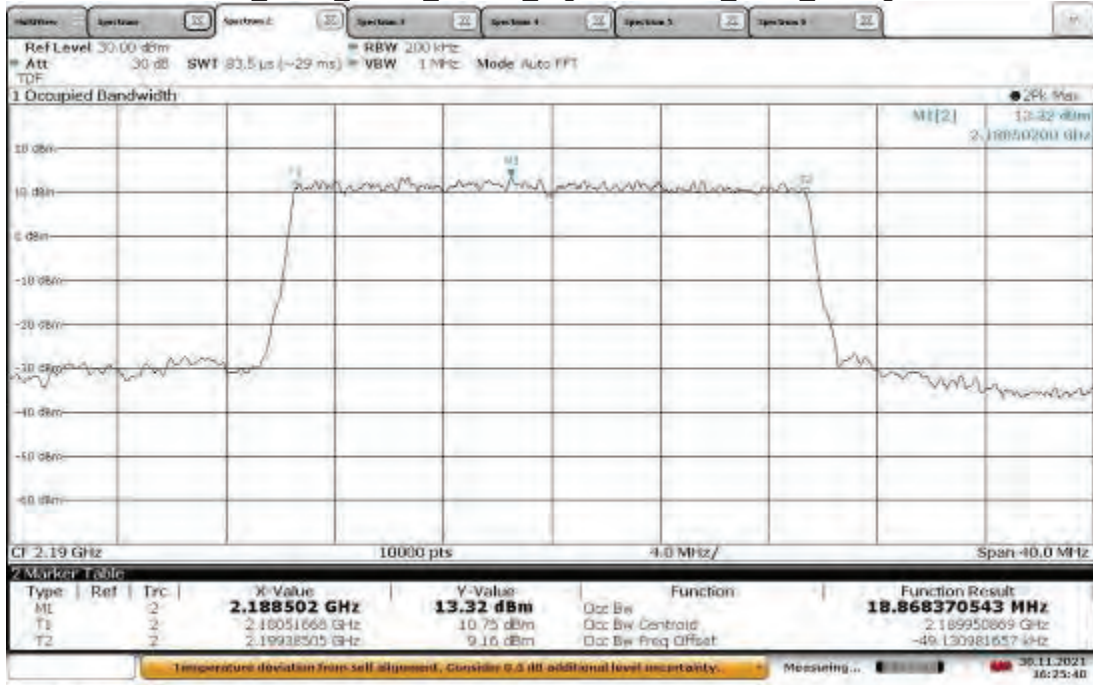
B66_ANT0_QPSK_20MHz_High 2190 MHz_OBW_20 deg
