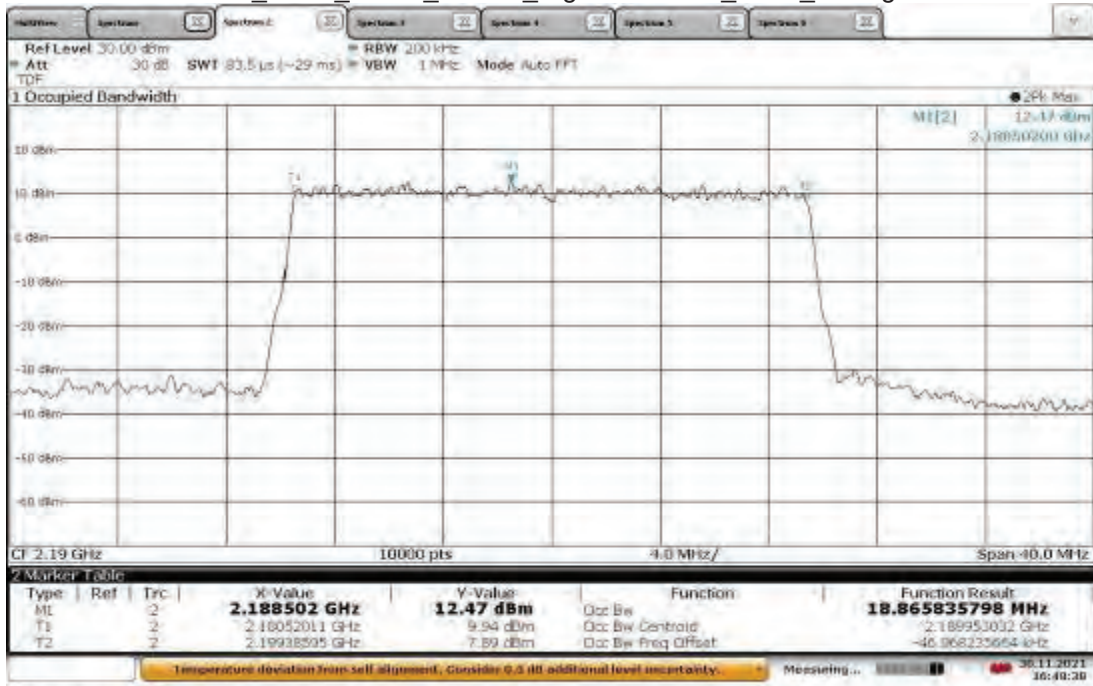
B66_ANT0_QPSK_20MHz_High 2190 MHz_OBW_30 deg
