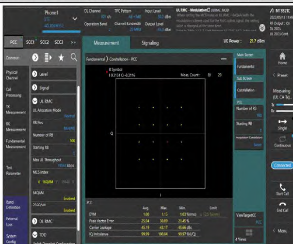
2-2-20MHz-20MHz-16QAM-16QAM-18801-18999-100RB#0-100RB#0
