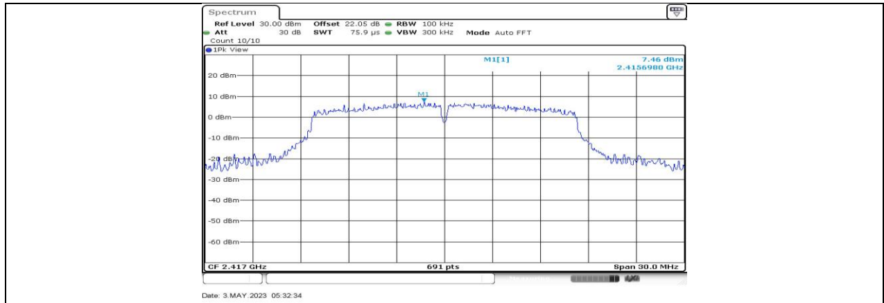
11G-CDD_Ant2_2417_0~Reference
