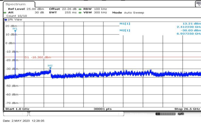
11B-CDD_Ant4_2412_1000~26500
