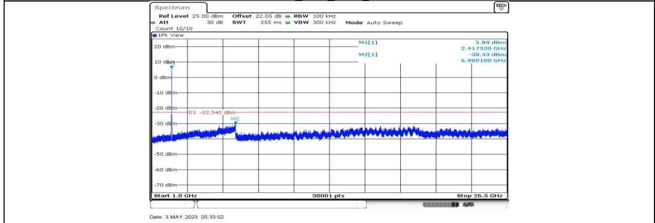
11G-CDD_Ant2_2417_1000~26500
