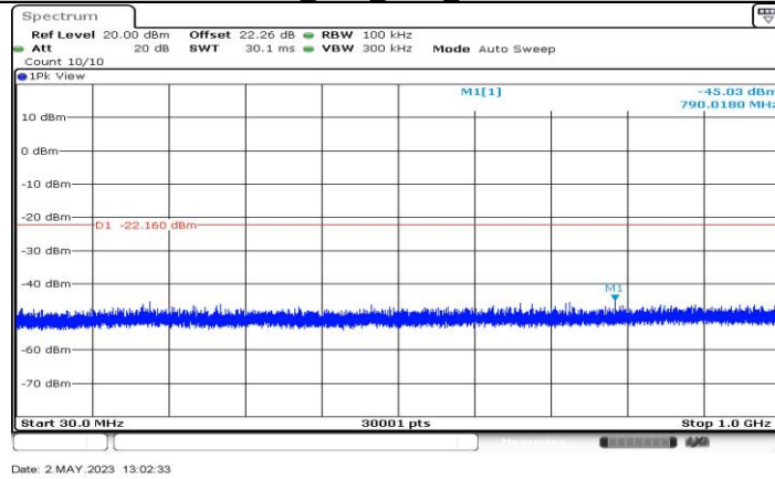
11G-CDD_Ant4_2412_30~1000
