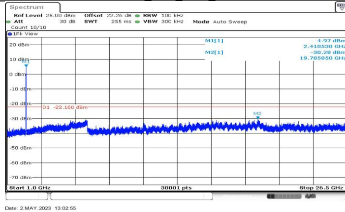
11G-CDD_Ant4_2412_1000~26500
