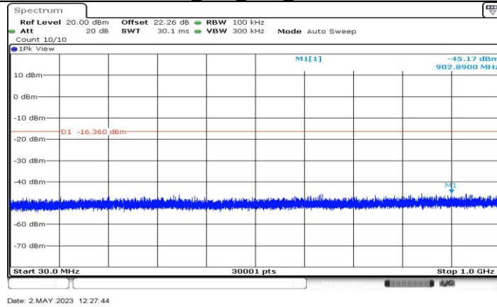
11B-CDD_Ant4_2412_30~1000
