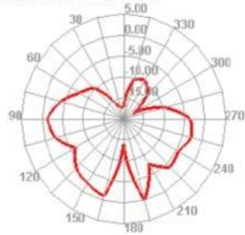
2450.000MHz E2
