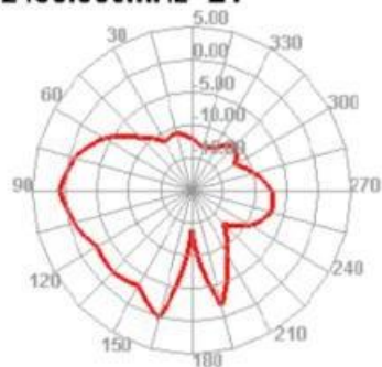
2450.000MHz E1
