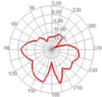
2500.000MHz E2
