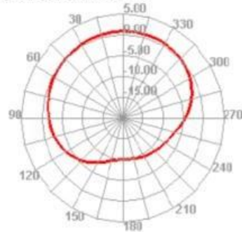
2500.000MHz H
