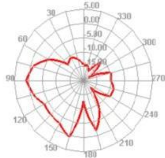
2500.000MHz E1
