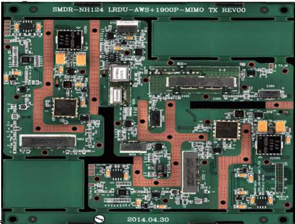
- SMT PCB TOP
