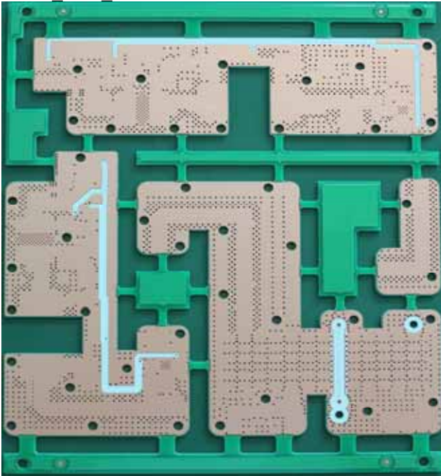
- Bare PAM PCB BOTTOM
