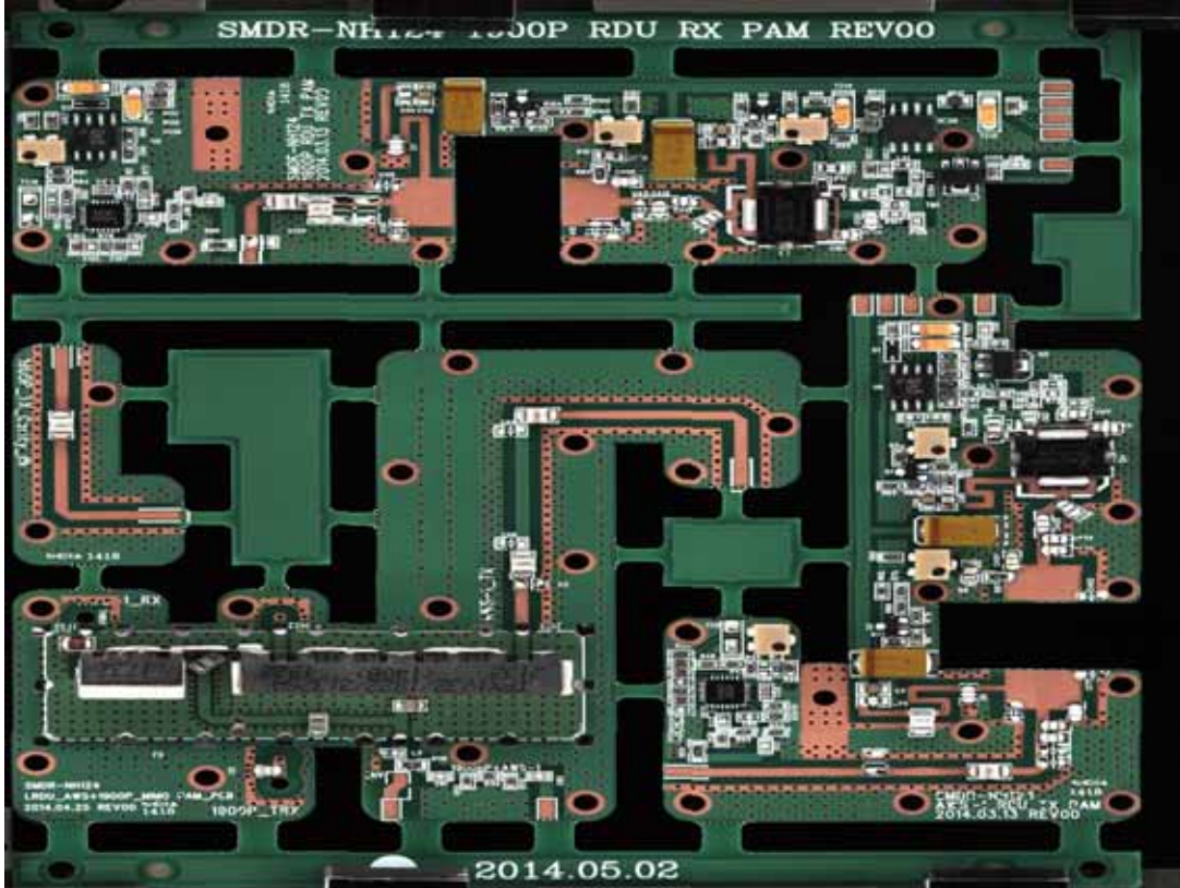
- SMT PCB TOP
