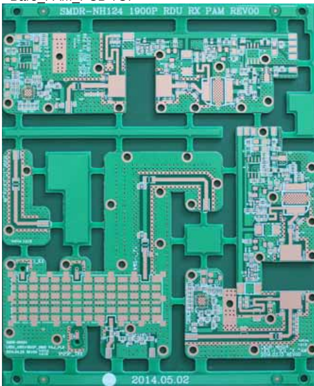
- Bare PAM PCB TOP
