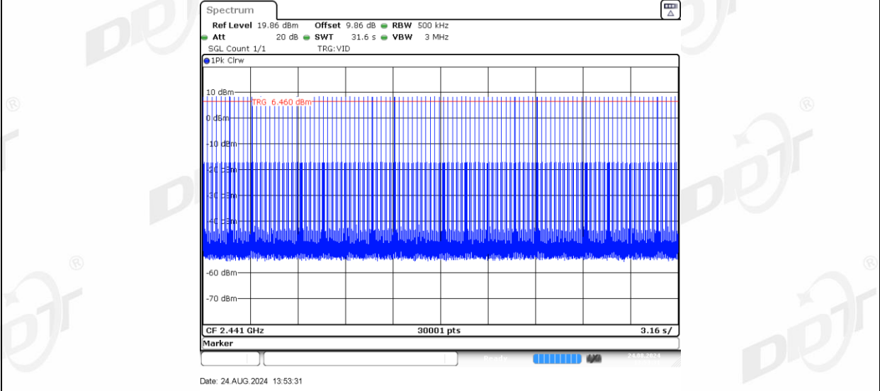
2DH1_Ant1_Hop
