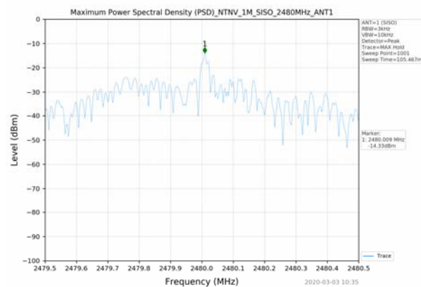
1M_2480MHz_SISO_ANT1
