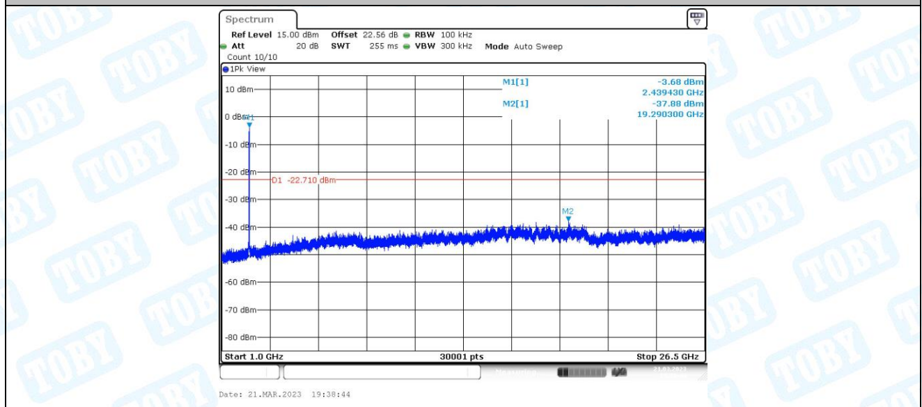
11N40MIMO_Ant2_2437_0~Reference
