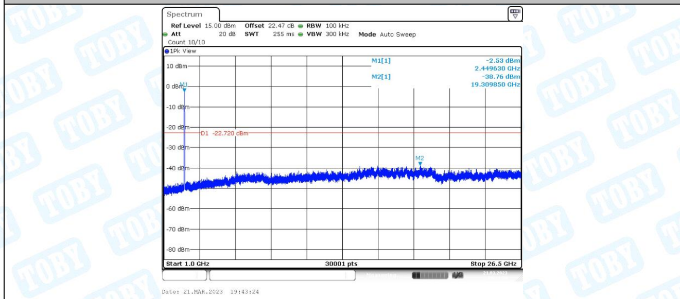
11N40MIMO_Ant2_2452_0~Reference
