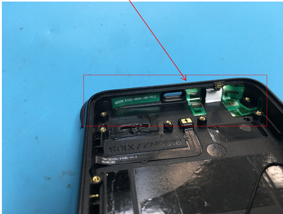
WWAN Main Antenna (GSM850/WCDMA B5/LTE B5/LTE B12 TX)
