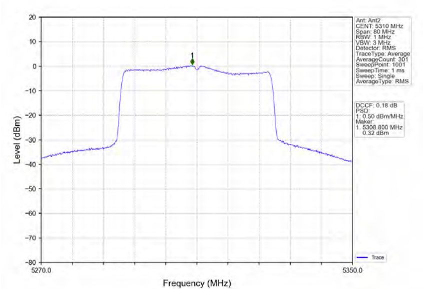
802.11ax(HEW40)_HCH_5310MHz_RU484_Left_Ant2_NTNV
