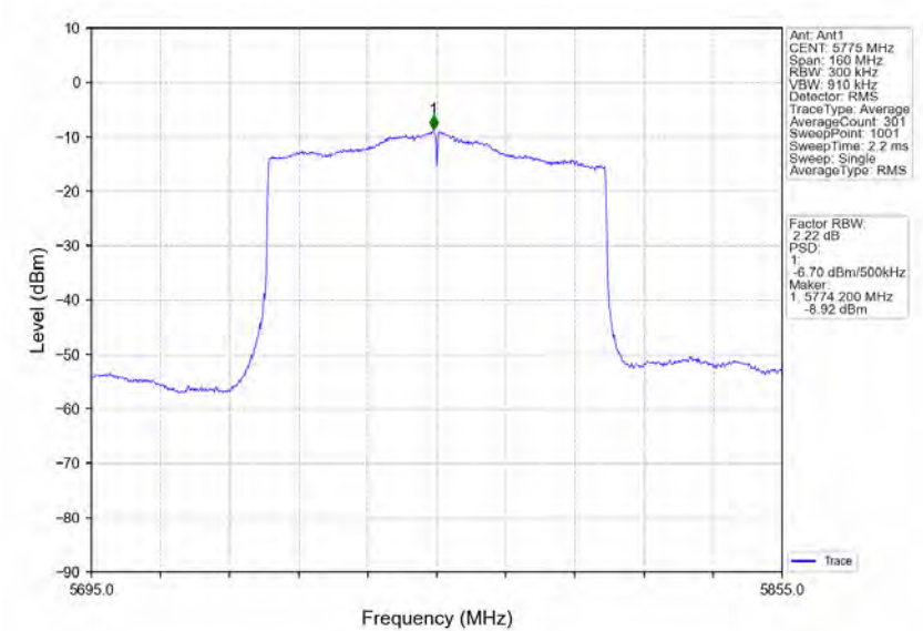
802.11ax(HEW80)_MCH_5775MHz_RU996_Left_Ant1_NTNV
