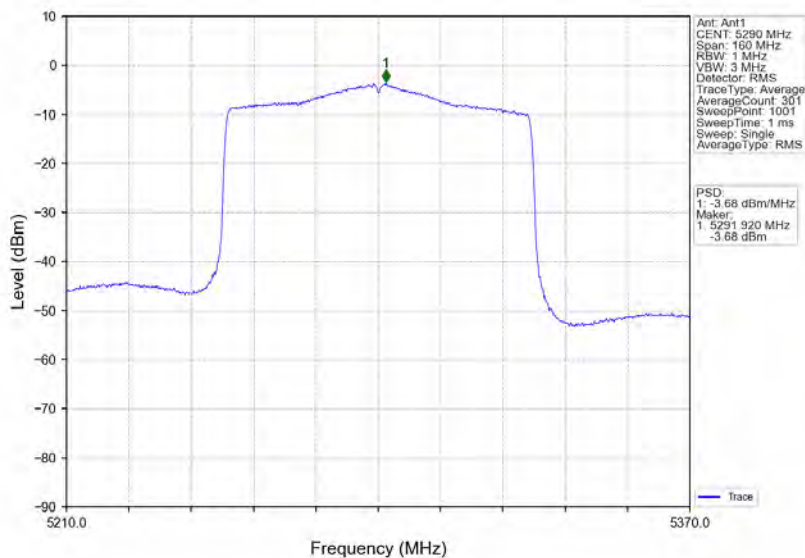
802.11ax(HEW80)_MCH_5290MHz_RU996_Left_Ant1_NTNV
