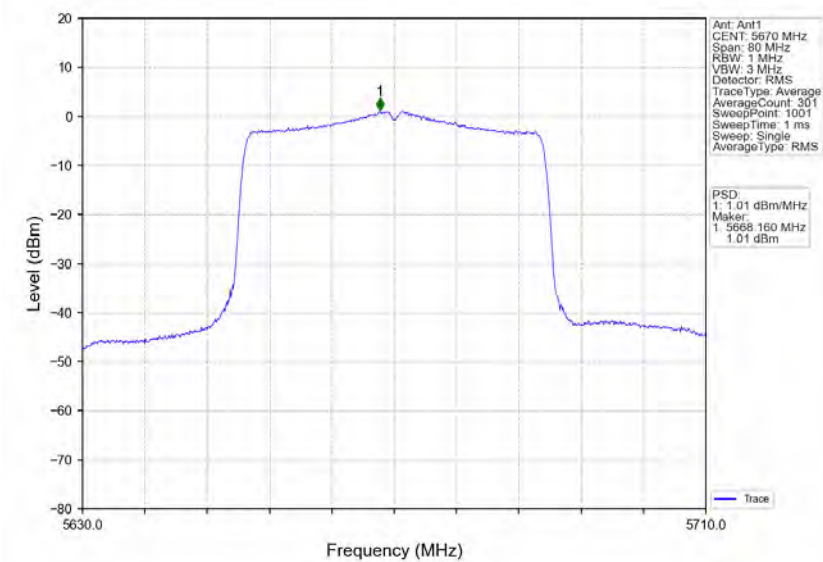
802.11ax(HEW40)_HCH_5670MHz_RU484_Left_Ant1_NTNV
