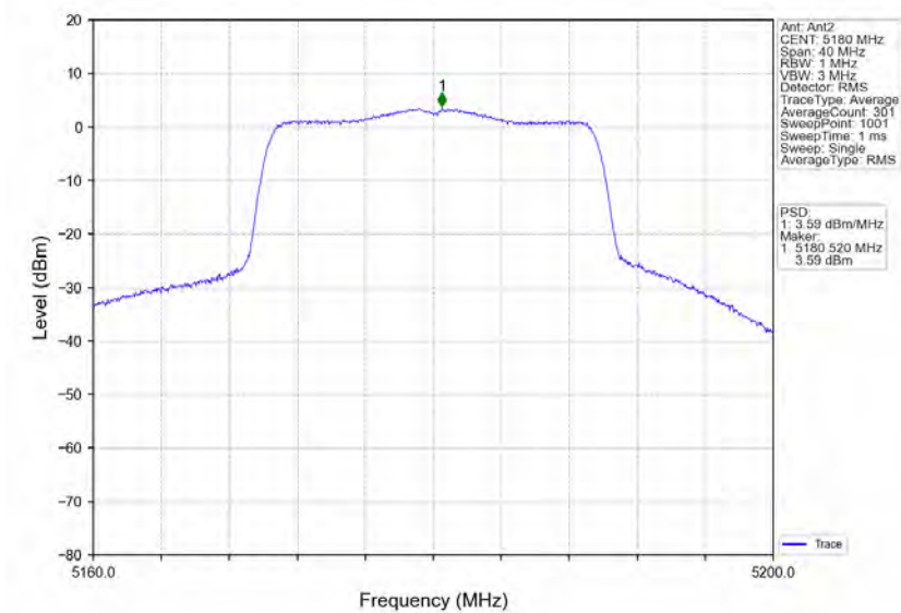
802.11ax(HEW20)_LCH_5180MHz_RU242_Left_Ant2_NTNV
