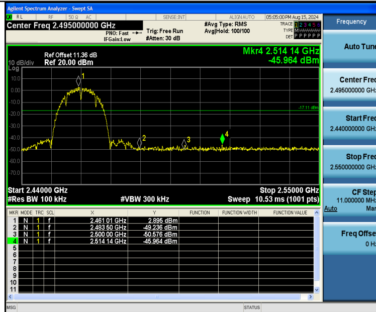
11B-Ant2-2462-PASS
