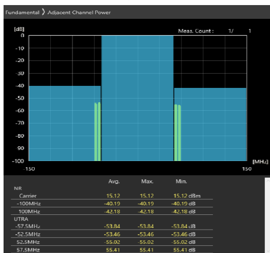
100MHz_30kHz_3650MHz-OFDM QPSK_RB135@67 -40.19,-42.18dB
