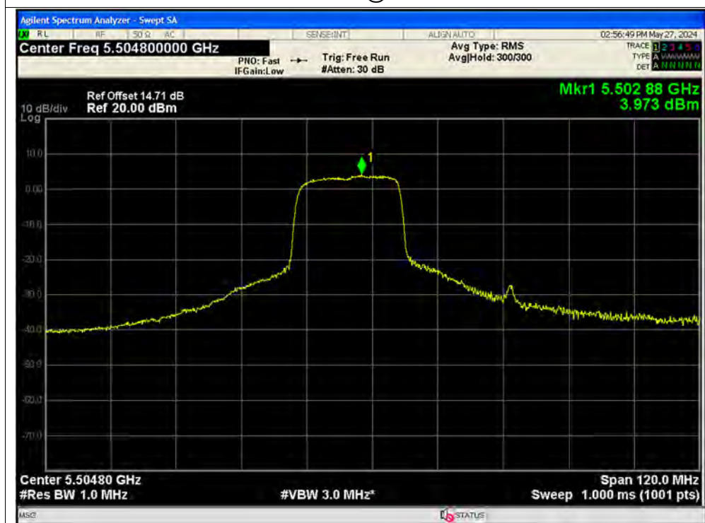
PSD NVNT ax80 242@61 5530MHz Ant1
