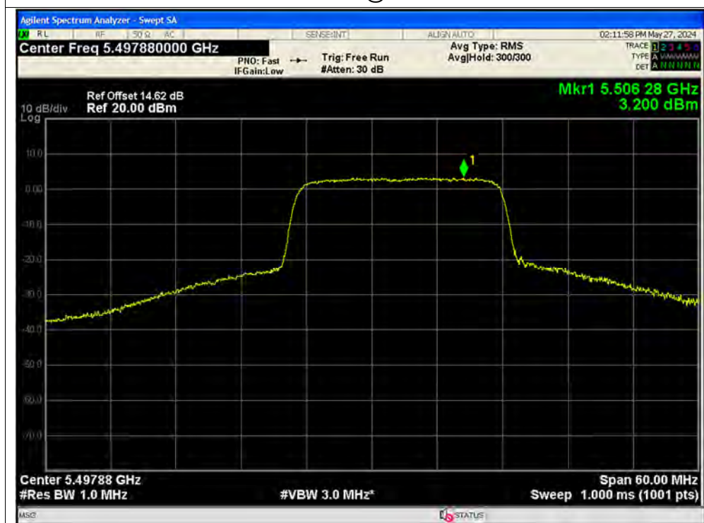
PSD NVNT ax40 242@61 5510MHz Ant1
