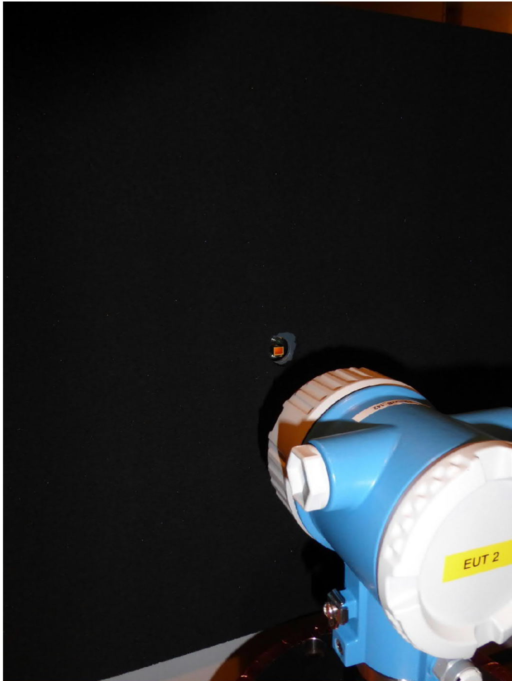
Test setup (>110 GHz)
